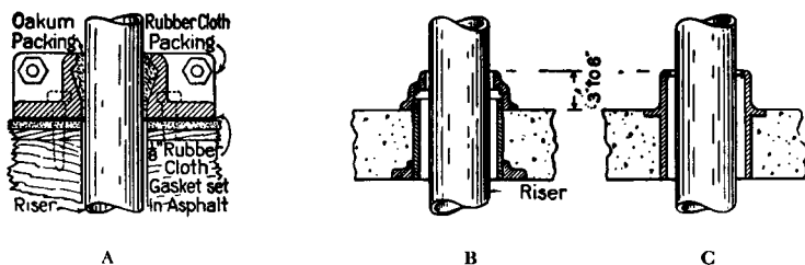
Fig. 3068. Watertight Riser Sleeves.
