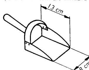
FIG. 2 — Hand-scoop
