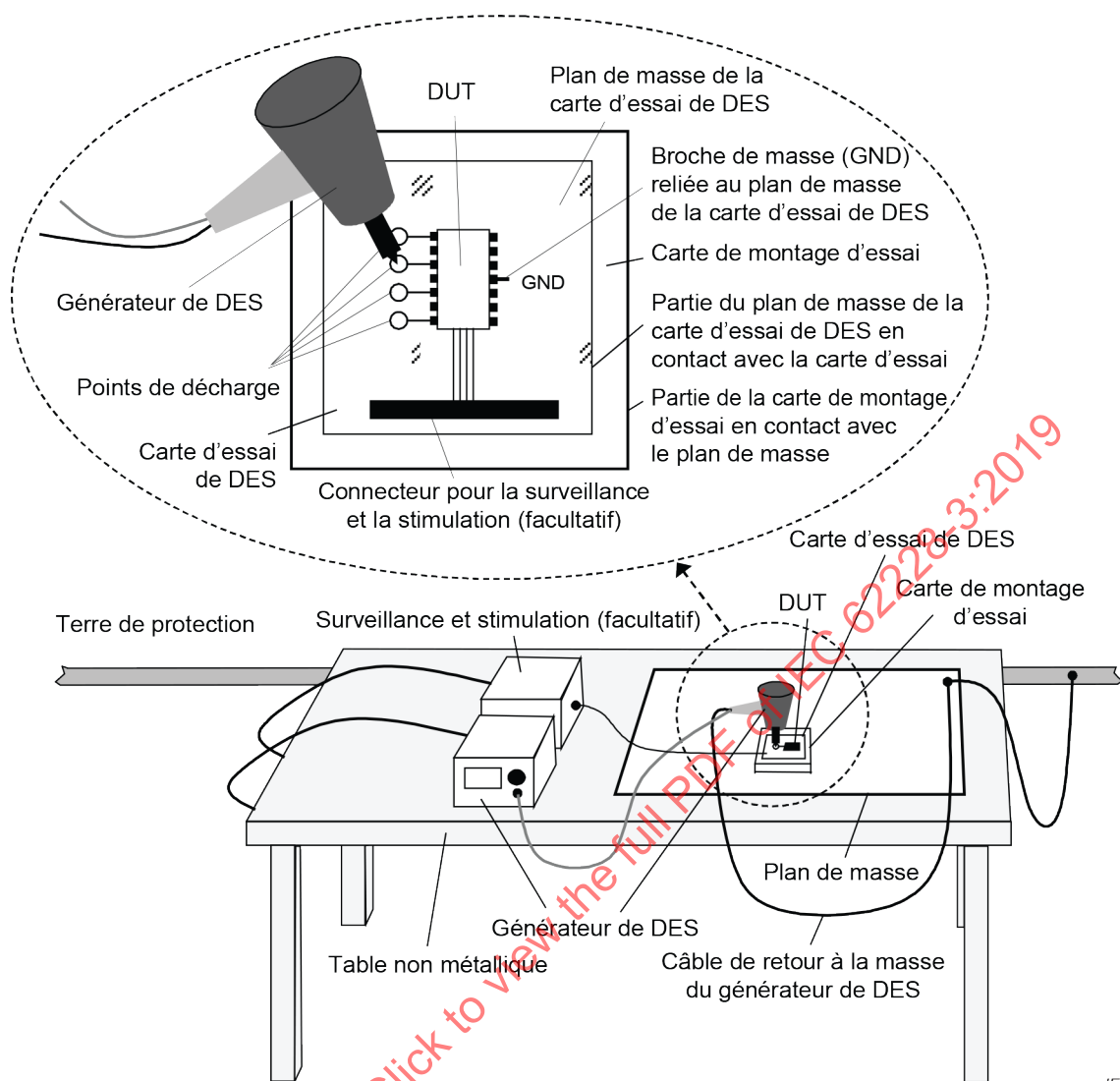
Figure 10 – Disposition d'essai pour les essais de décharge électrostatique directe – Disposition principale
