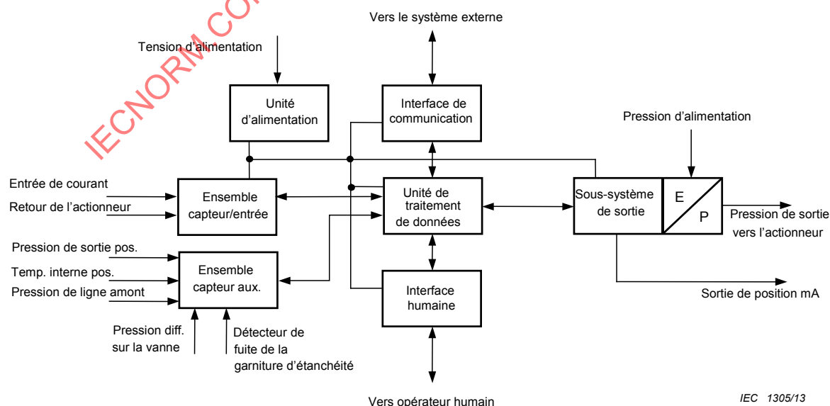
Figure 1 – Modèle de positionneur en configuration étendue
