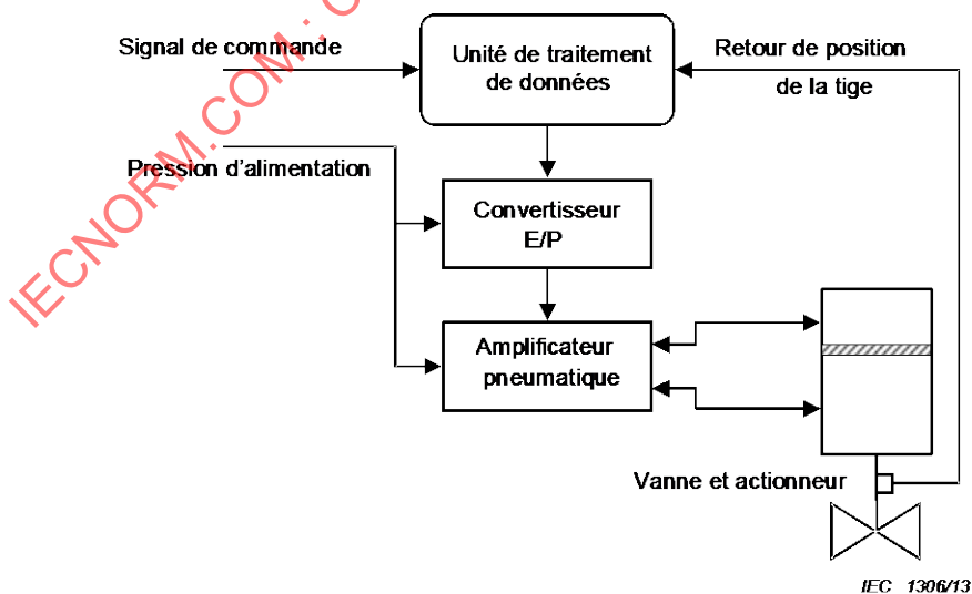
Figure 2 – Conception de base pour des positionneurs à sorties analogiques
