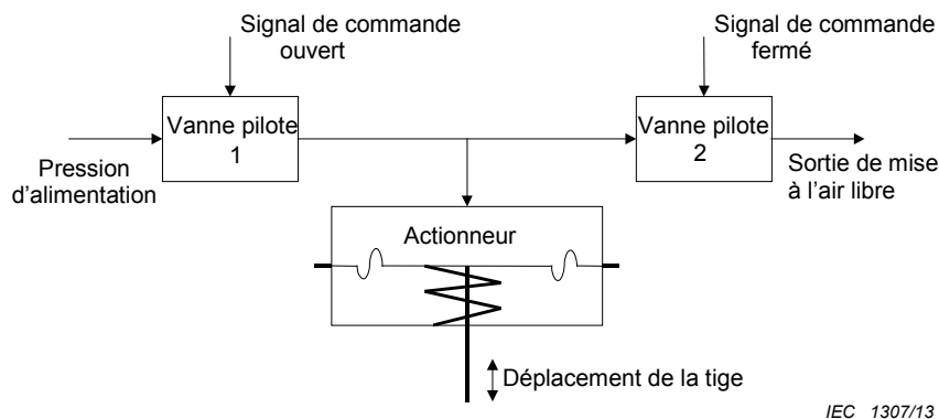
Figure 3 – Conception de base pour des positionneurs à sortie pulsée
