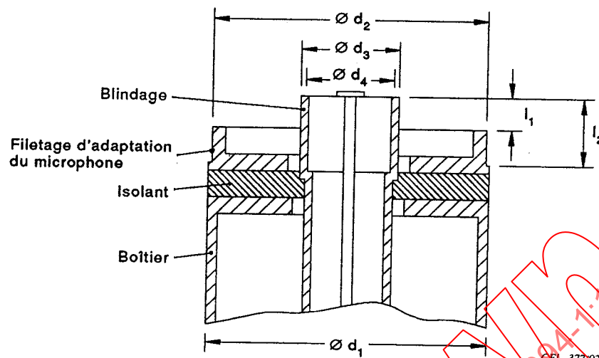
Figure 2 – Fixation mécanique du microphone montrant la configuration de référence du blindage
