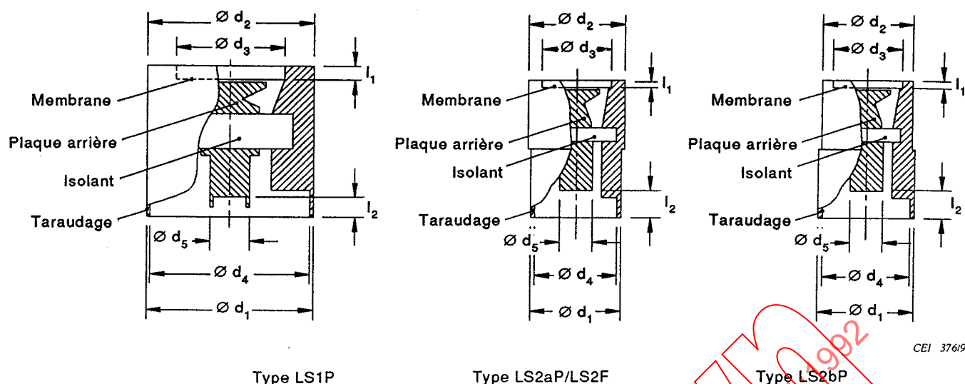
Figure 1 – Configurations mécaniques des microphones
