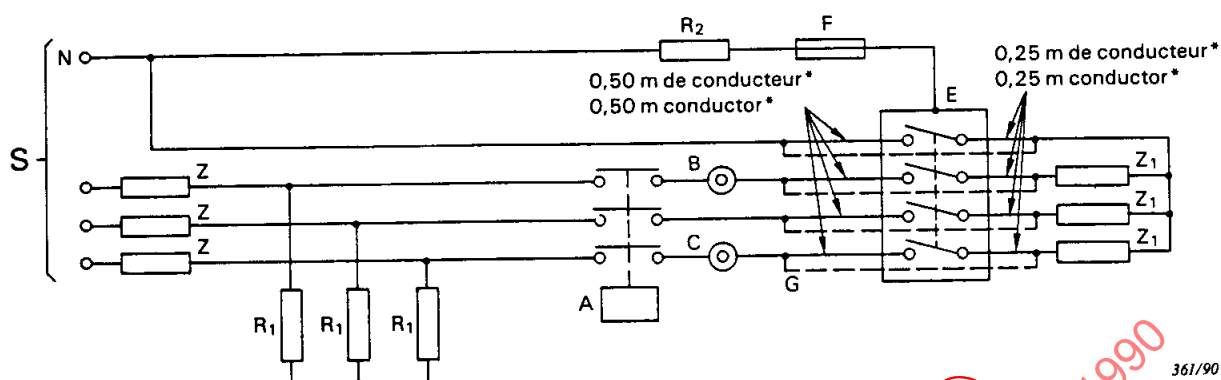
Figure 6 - Disjoncteur tétrapolaire Four-pole circuit-breaker
