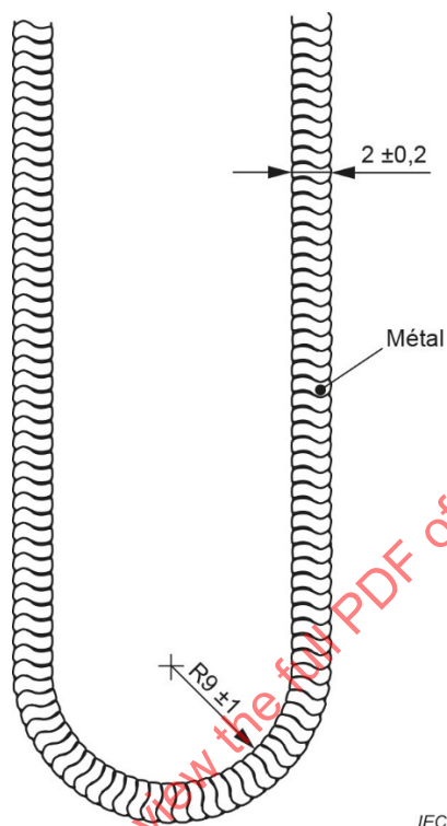
Figure 35 – Chaîne d'essai
