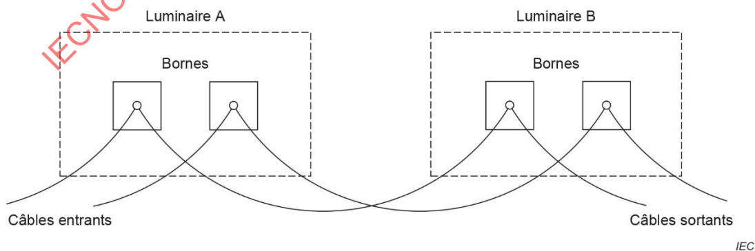
Figure 1 – Exemple de "repiquage" (passage en coupure)
