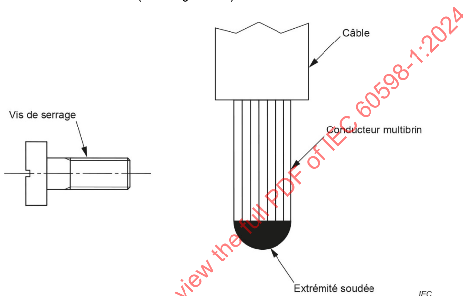
Figure 36 – Exemple de degré d'étamage admis
