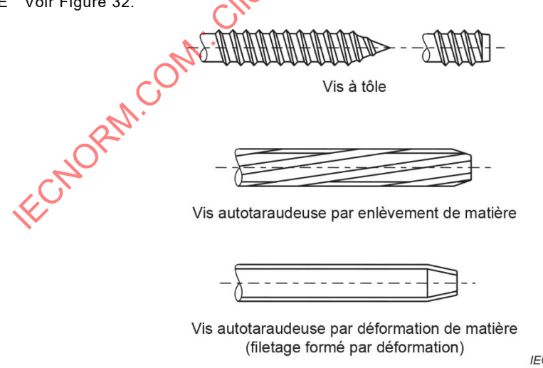
Figure 32 – Exemples de vis à tôle et de vis autotaraudeuses par enlèvement ou déformation de matière
