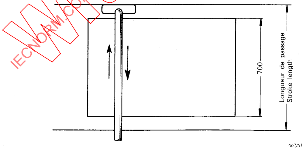
FIG. 2. — Longueur de passage pour les mesures de dépoussiérage et de ramassage des fils. Stroke length in the dust removal and thread removal measurements.
