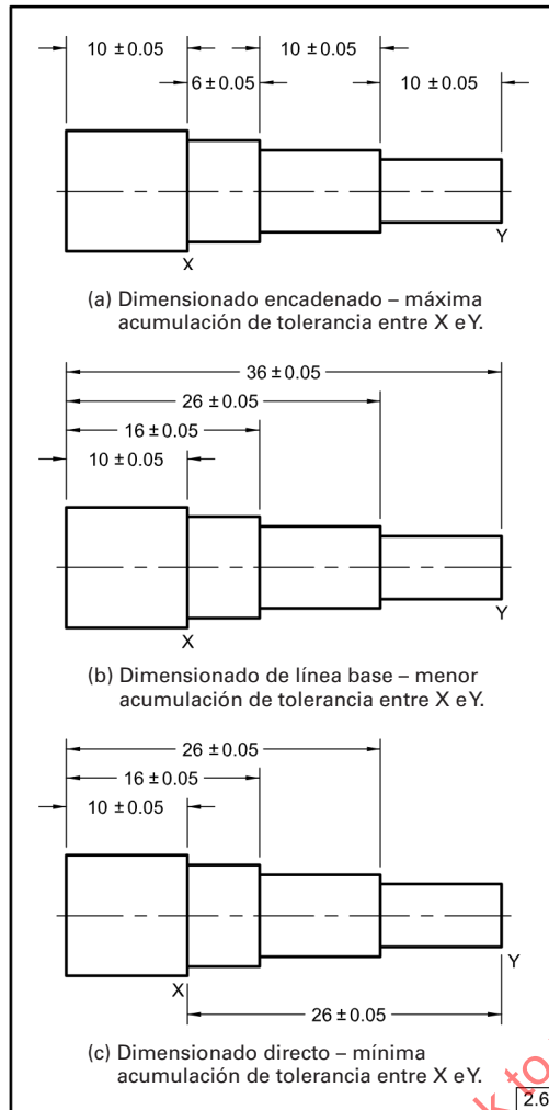
Fig. 2-4 Acumulación de tolerancias
