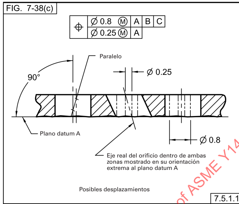
Fig. 7-38 Patrón de Orificios Localizados por Tolerancia Compuesta de Posición (Continuación) (Zonas de Tolerancia para Patrón de Orificios)
