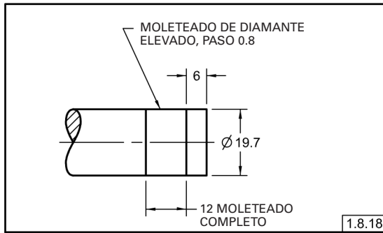
Fig. 1-47 Moleteados
