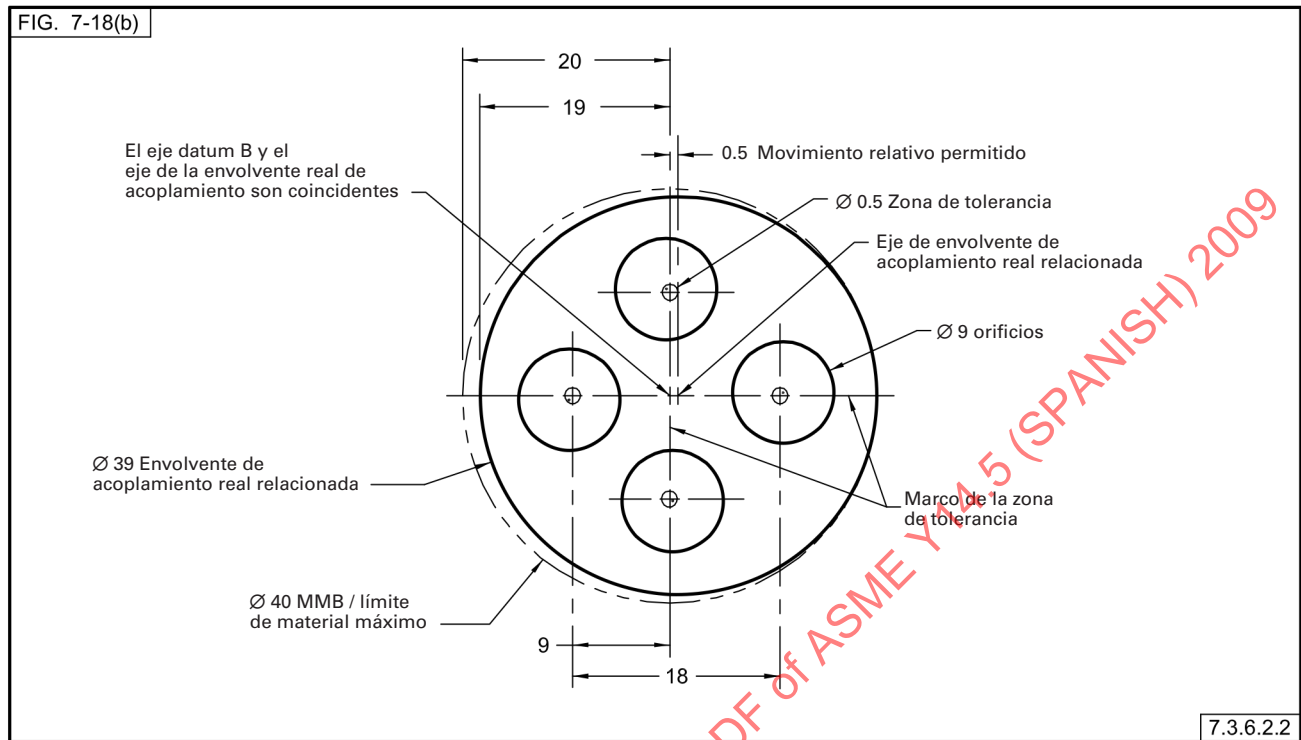
Fig. 7-18 Elemento Datum Referenciado a MMB (Continuación)
