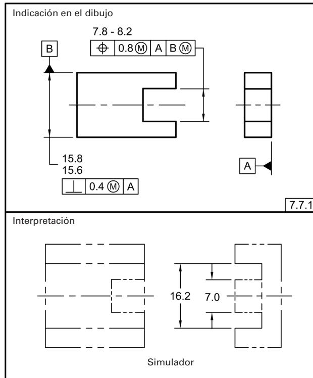
Fig. 7-64 Tolerancia de Posición a MMC para Elementos Simétricos
