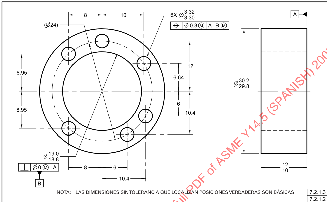
Fig. 7-2 Tolerancia de Posición con Datums de Referencia
