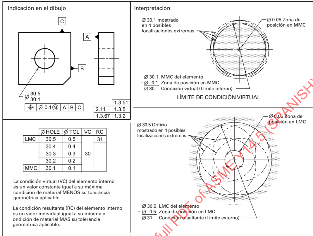
Fig. 2-12 Límites de Condición Virtual y Resultante Usando el Concepto MMC – Elemento Interno
