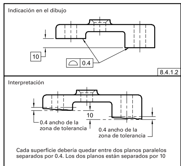
Fig. 8-16 Especificación del Perfil de una Superficie para Superficies Escalonadas
