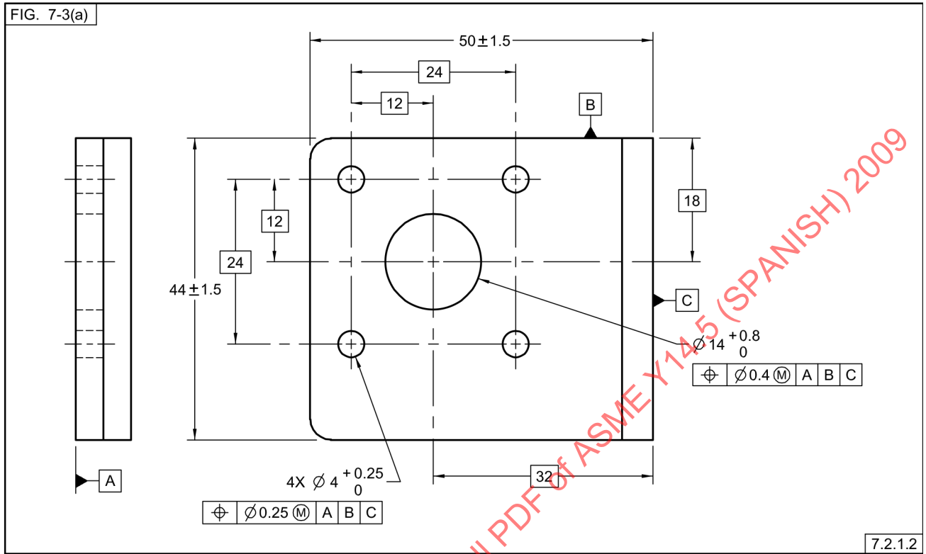
Fig. 7-3 Tolerancia de Posición en Relación con Planos de Superficies de Elementos Datum
