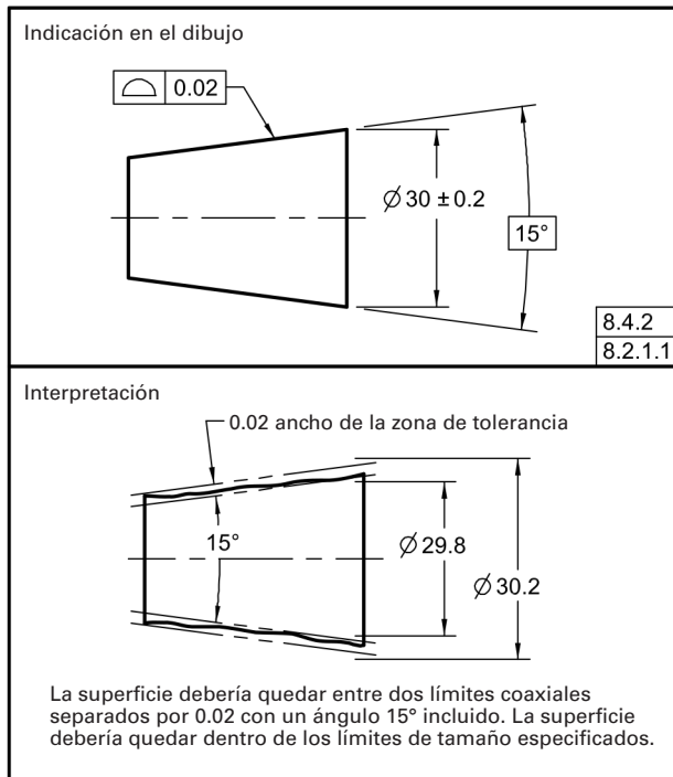
Fig. 8-17 Especificación del Perfil de un Elemento Cónico
