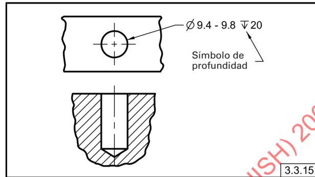
Fig. 3-17 Símbolo de Profundidad
