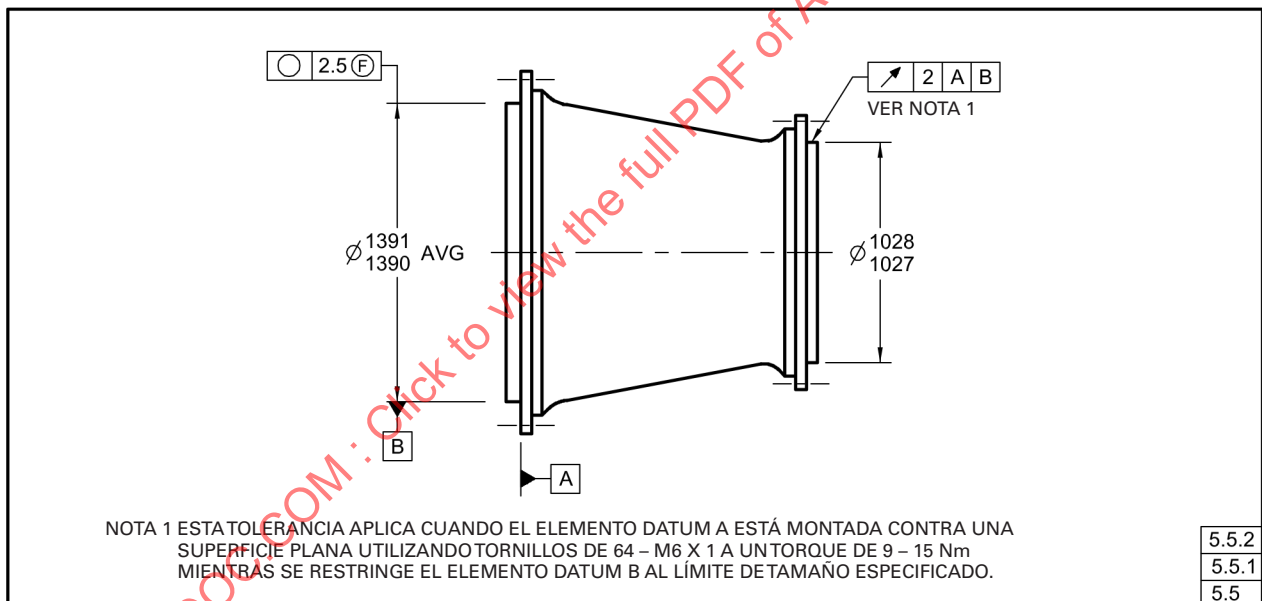
Fig. 5-14 Especificación de la Restricción para Piezas No Rígidas
