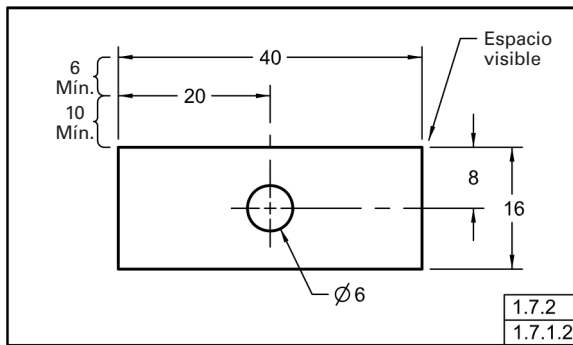
Fig. 1-8 Espaciamiento de Líneas de Dimensión
