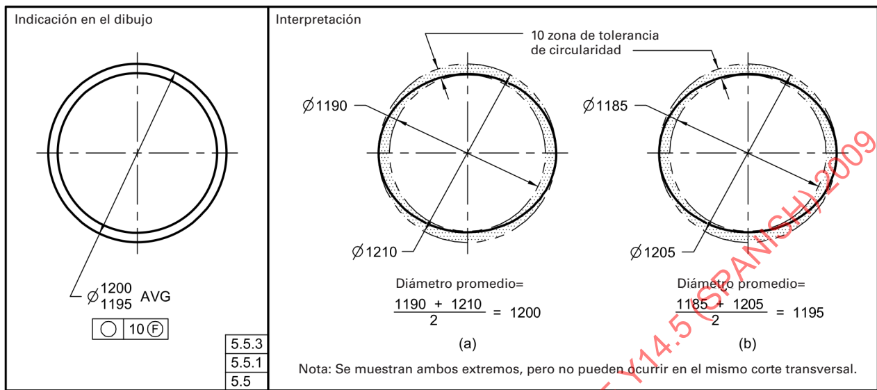
Fig. 5-13 Especificación de la Circularidad en Estado Libre con Diámetro Promedio
