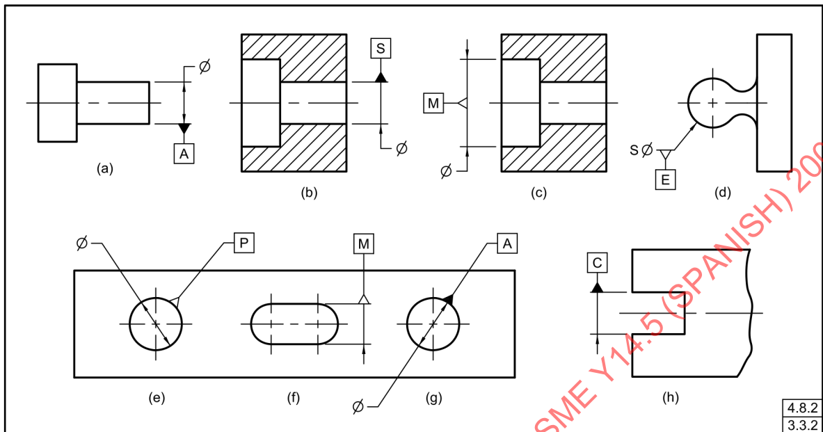
Fig. 3-4 Localización de Símbolos de Elementos Datum en Elementos de Tamaño
