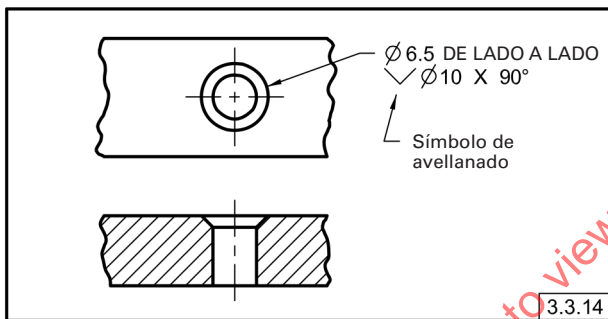
Fig. 3-16 Símbolo de Avellanado
