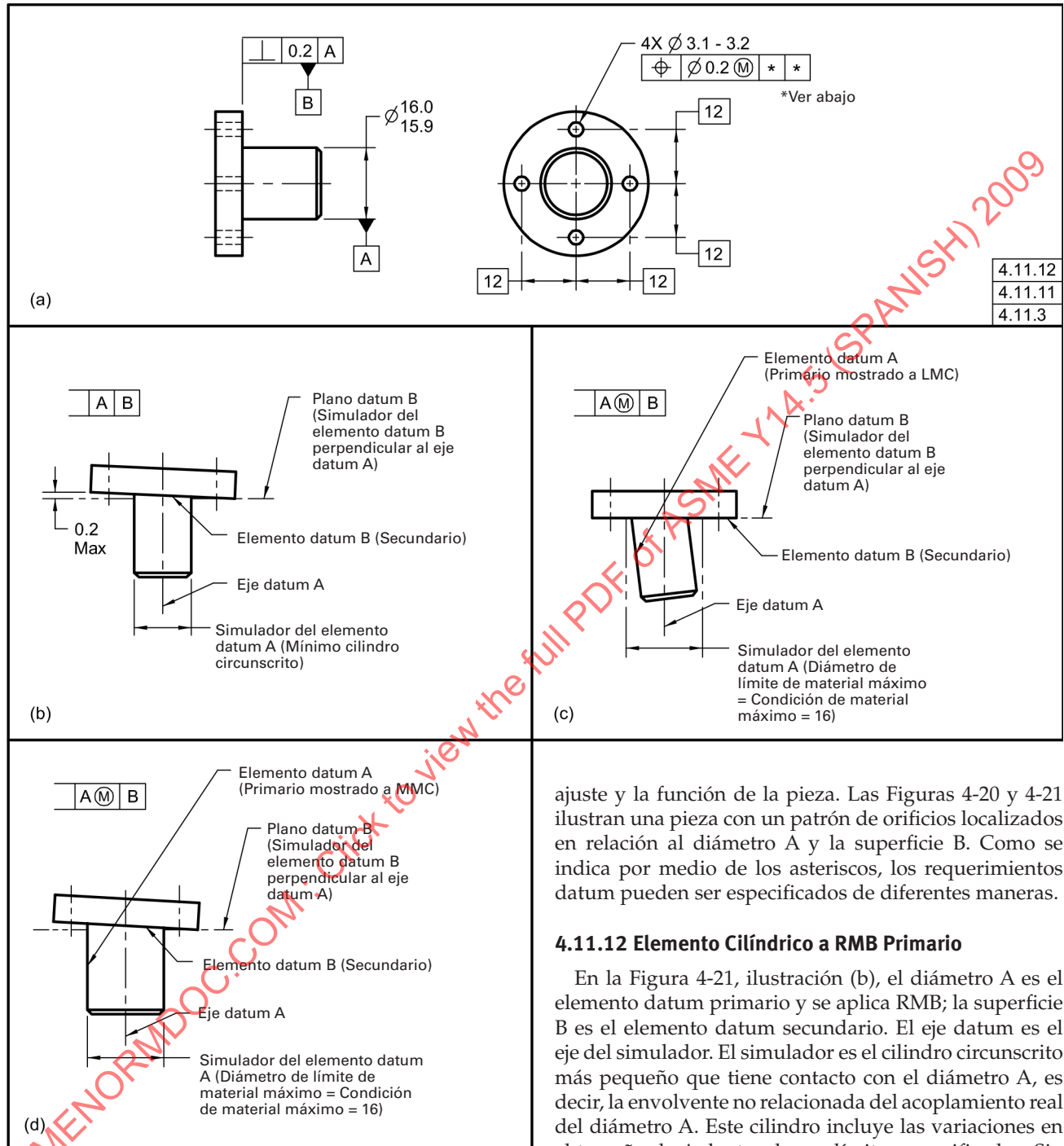
Fig. 4-21 Efecto de la Condición de Material
