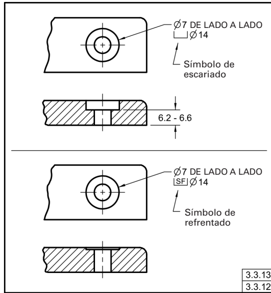
Fig. 3-15 Símbolos de Escariado o Refrentado
