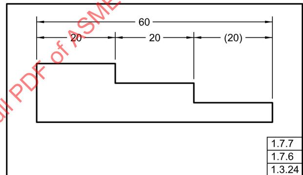
Fig. 1-19 Dimensión de Referencia Intermedia
