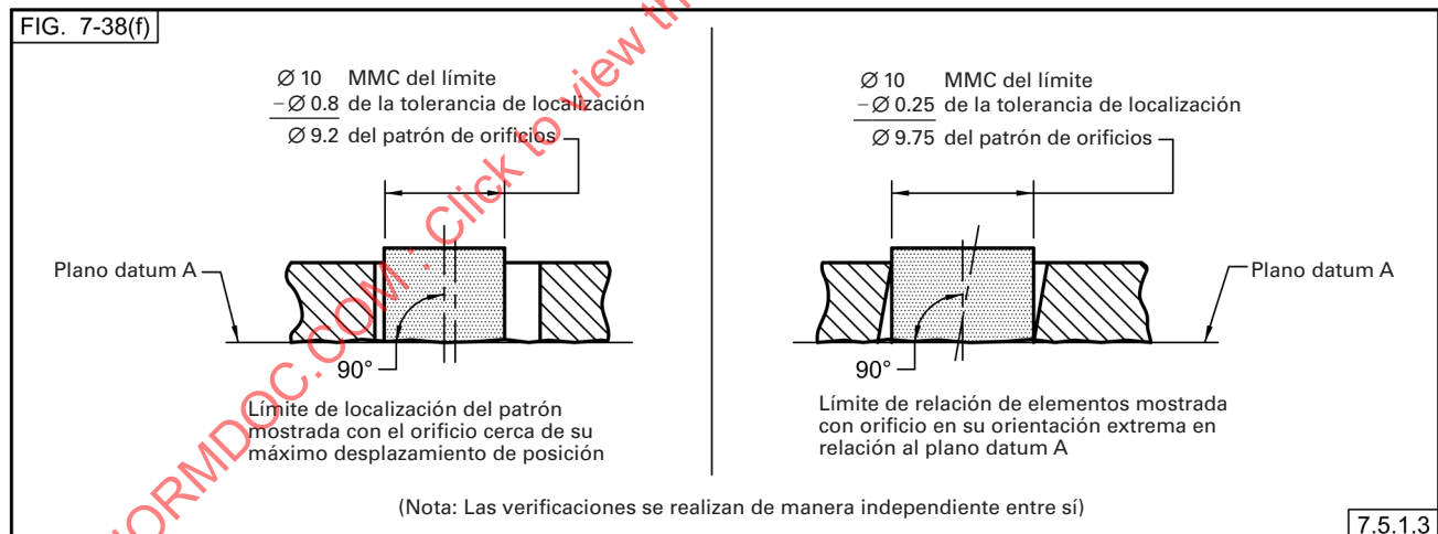
Fig. 7-38 Patrón de Orificios Localizados por Tolerancia Compuesta de Posición (Continuación) (Límites de Aceptación de Orificios en Patrones)
