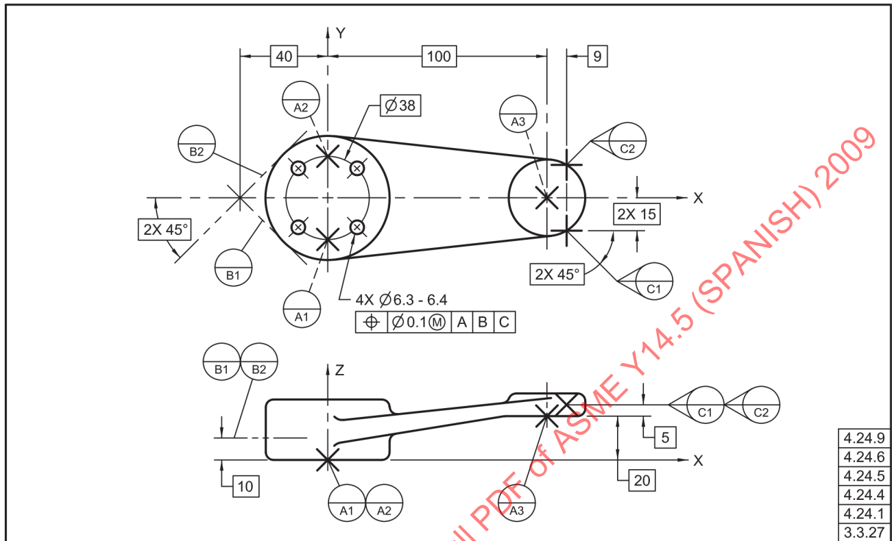
Fig. 4-47 Aplicación de Datums Móviles
