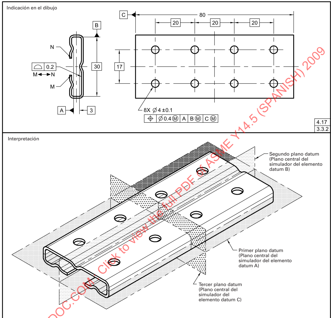
Fig. 4-33 Elementos de Tamaño Regular e Irregular como Elementos Datum
