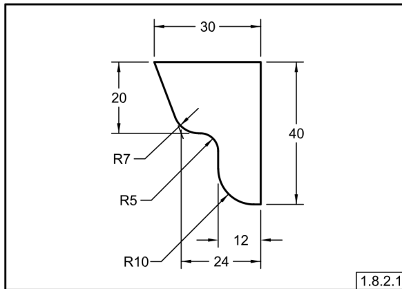
Fig. 1-24 Radios con Centros No Localizados
