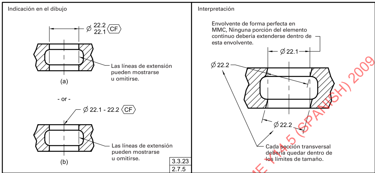
Fig. 2-9 Elemento Continuo, Cilíndrico Interno
