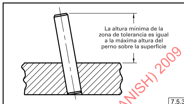
Fig. 7-23 Zona de Tolerancia Proyectada Aplicada a Espárragos o Pasadores
