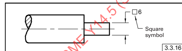
Fig. 3-18 Símbolo de Cuadrado
