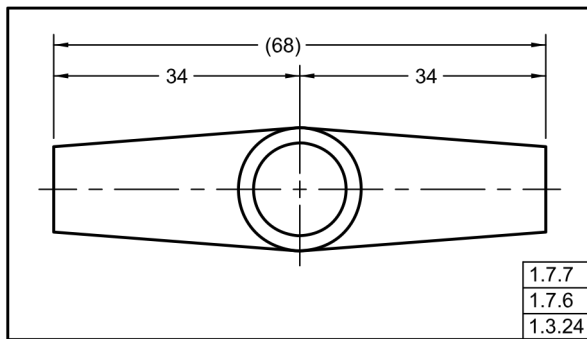
Fig. 1-20 Dimensión de Referencia Total
