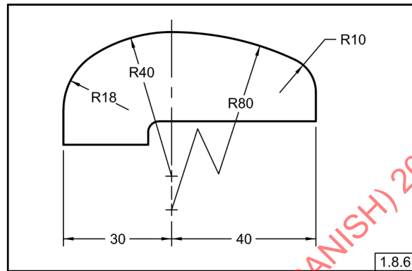
Fig. 1-32 Contorno de Arco Circular
