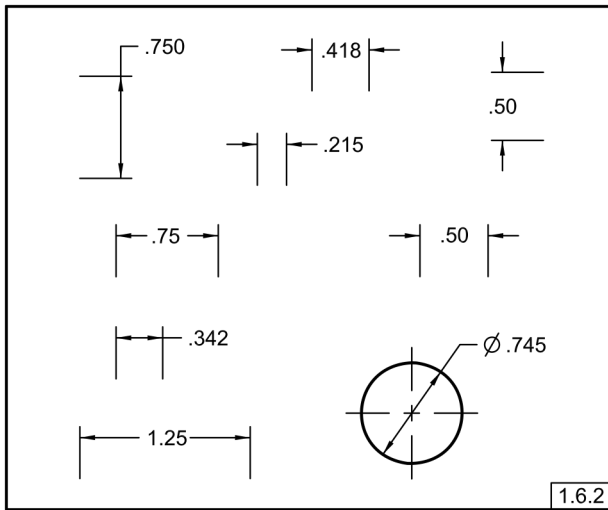
Fig. 1-5 Dimensiones en Pulgadas Decimales
