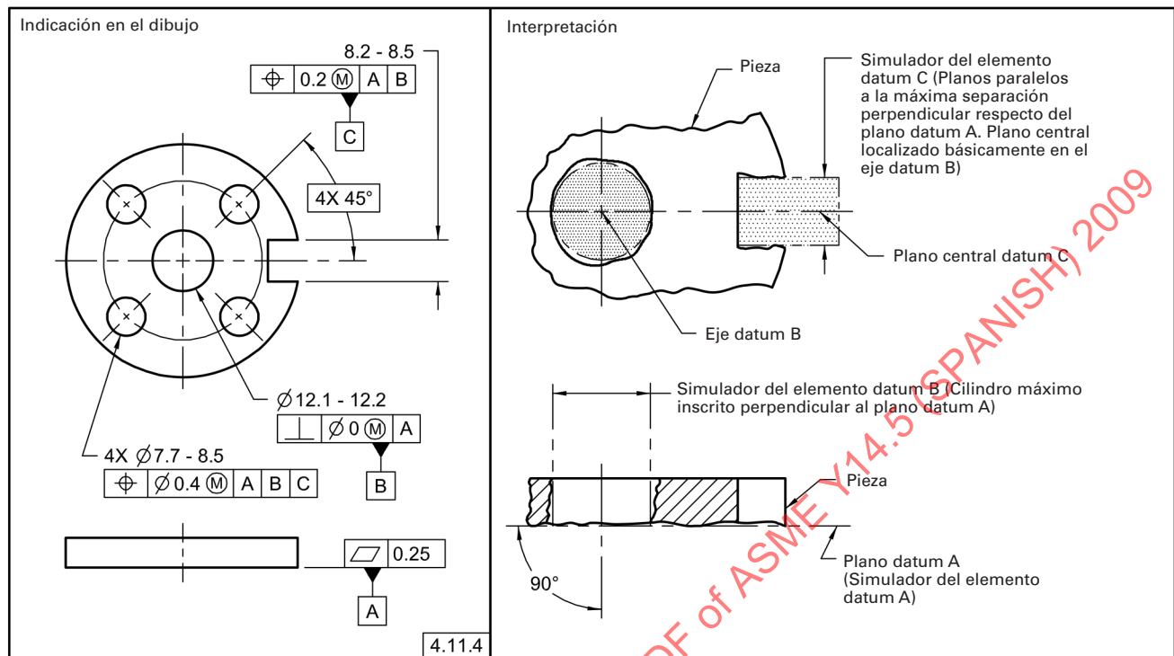
Fig. 4-15 Elementos Datum Secundario y Terciario – RMB
