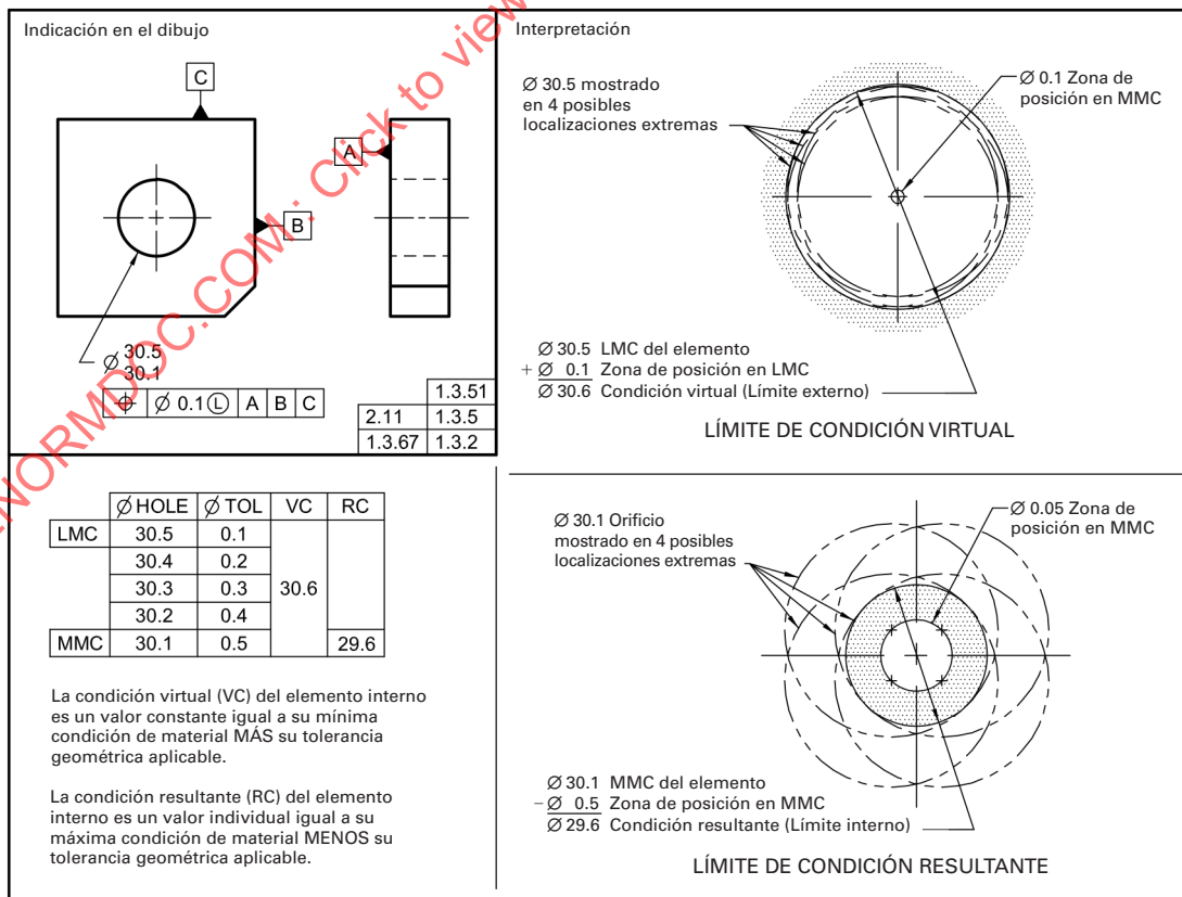
Fig. 2-13 Límites de Condición Virtual y Resultante Usando el Concepto LMC – Elemento Interno
