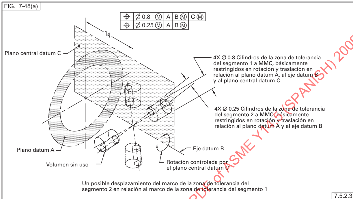
Fig. 7-48 Patrón Radial de Orificios Localizado por Marcos de Control de Elemento de Múltiples Segmentos Individuales (Continuación) (Zonas de Tolerancia para Patrón Radial de Orificios)
