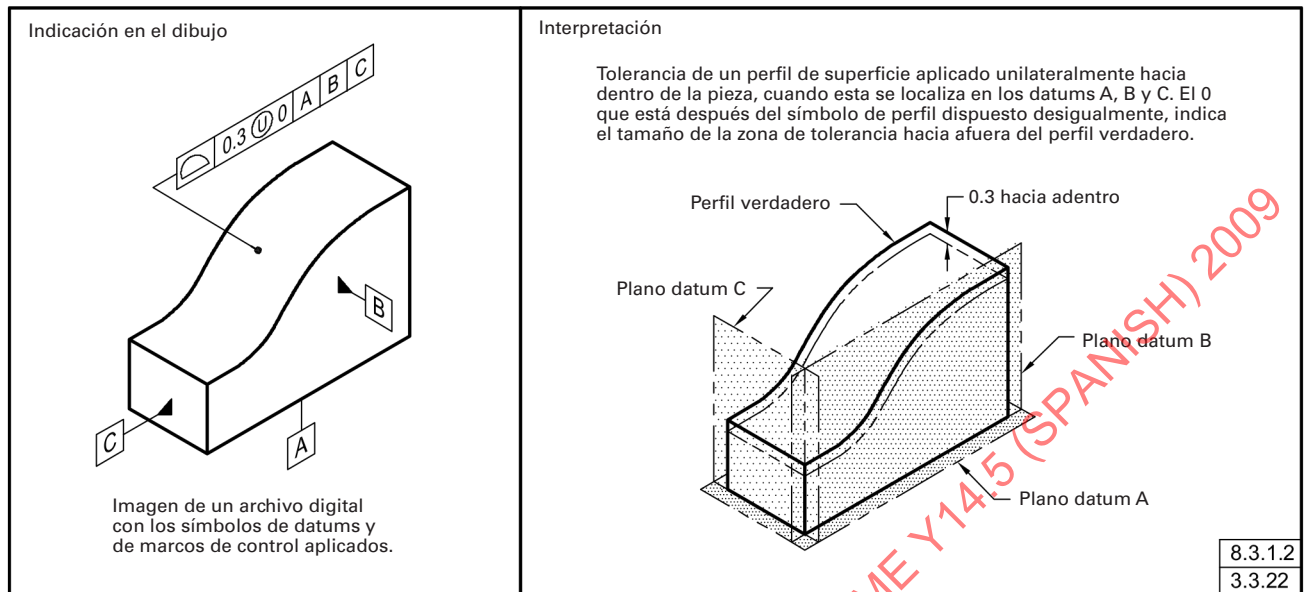
Fig. 8-2 Aplicación 3D de un Perfil de Superficie (Interno Unilateralmente)
