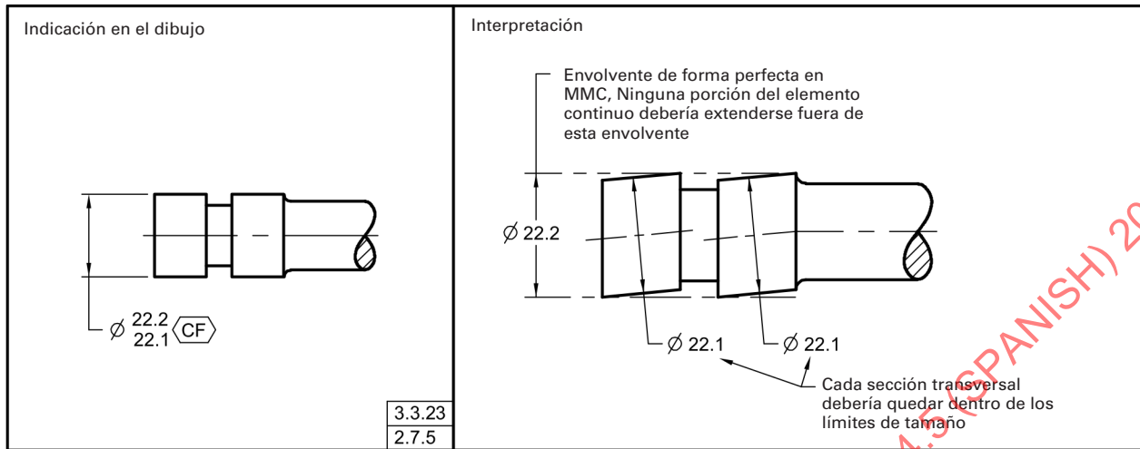
Fig. 2-8 Elemento Continuo, Cilíndrico Externo
