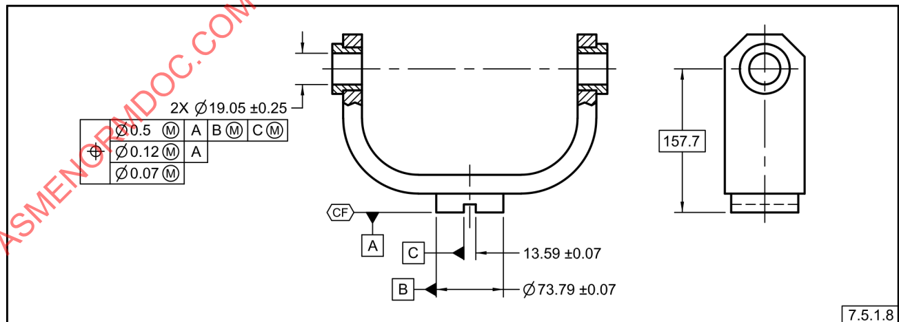
Fig. 7-45 Tolerancia Compuesta de Tres Segmentos
