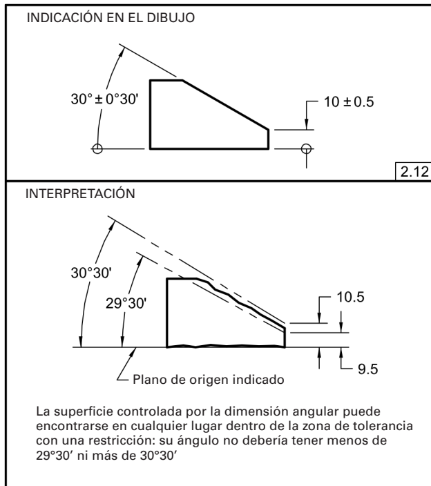
Fig. 2-18 Tolerancia de una Superficie Angular Usando una Combinación de Dimensiones Lineales y Angulares
