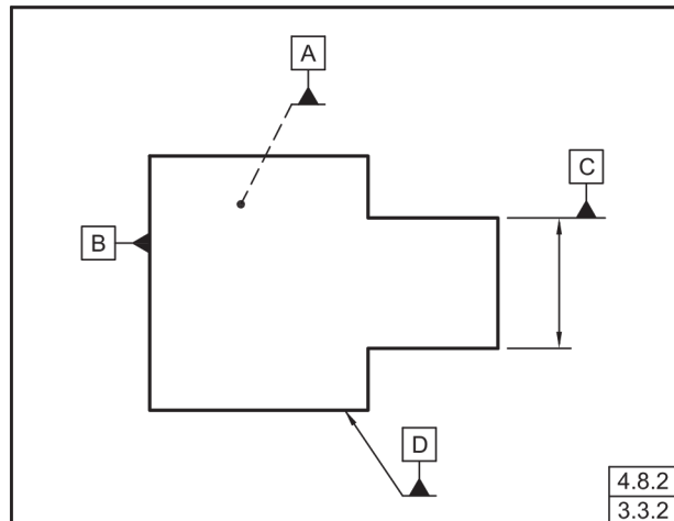
Fig. 3-3 Símbolos de Elementos Datum en una Superficie de Elemento y una Línea de Extensión
