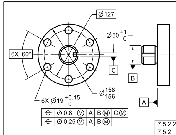
Fig. 7-47 Tolerancia de Posición con Marcos de Control de Elemento de Múltiples Segmentos Individuales
