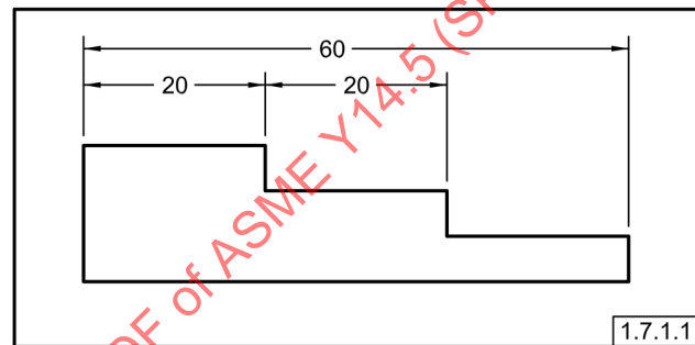
Fig. 1-7 Agrupamiento de Dimensiones
