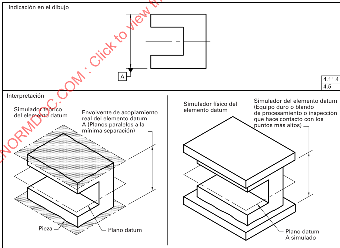
Fig. 4-13 Establecimiento de Datums – Para Ancho de Datum Externo – RMB
