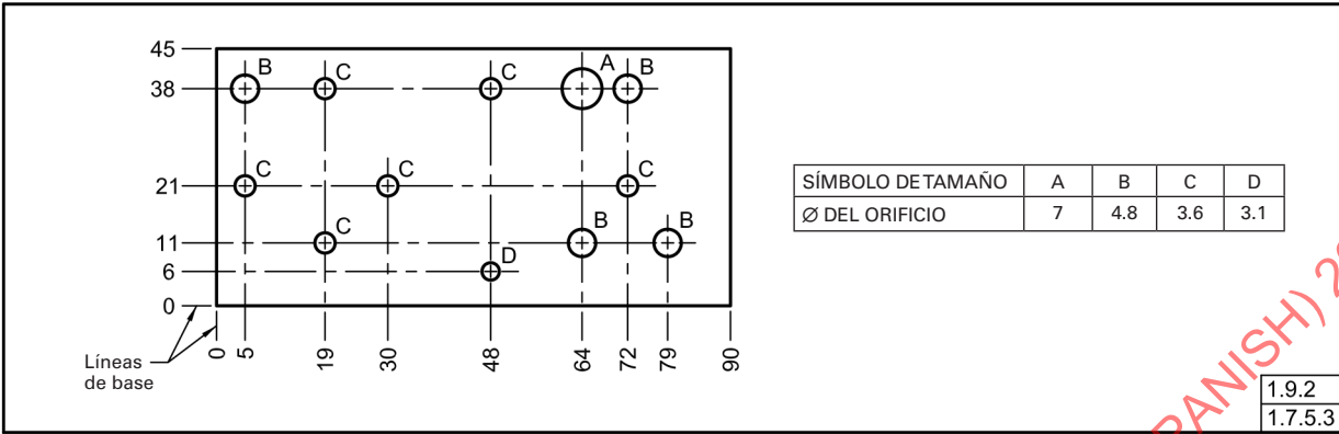
Fig. 1-51 Dimensionado por Coordenadas Rectangulares en Forma Tabular
