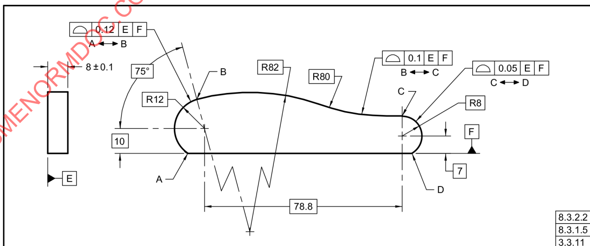
Fig. 8-6 Especificación de Diferentes Tolerancias en los Segmentos de un Perfil
