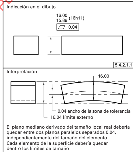
Fig. 5-8 Especificación de la Planicidad de un Plano Medio Derivado – RFS
