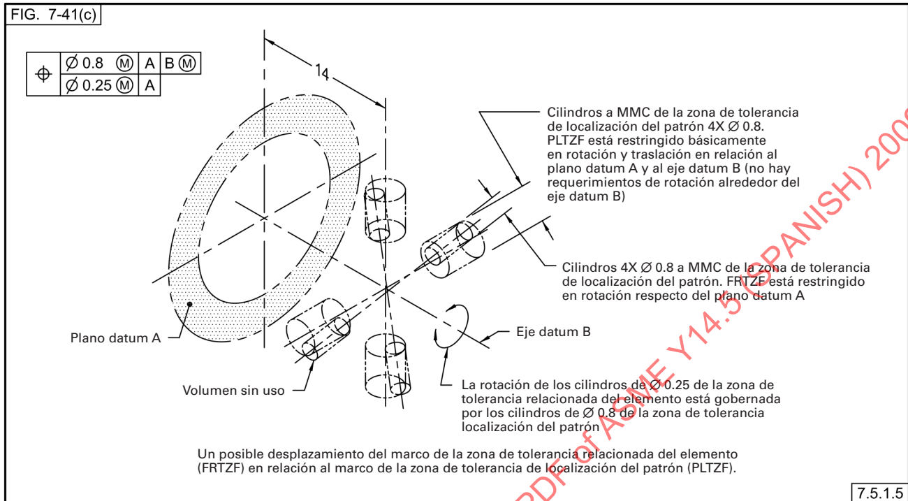
Fig. 7-41 Patrón Radial de Orificios Localizado por medio de Tolerancia Compuesta de Posición (Continuación) (Zonas de Tolerancia para Patrones Radiales de Orificios)
