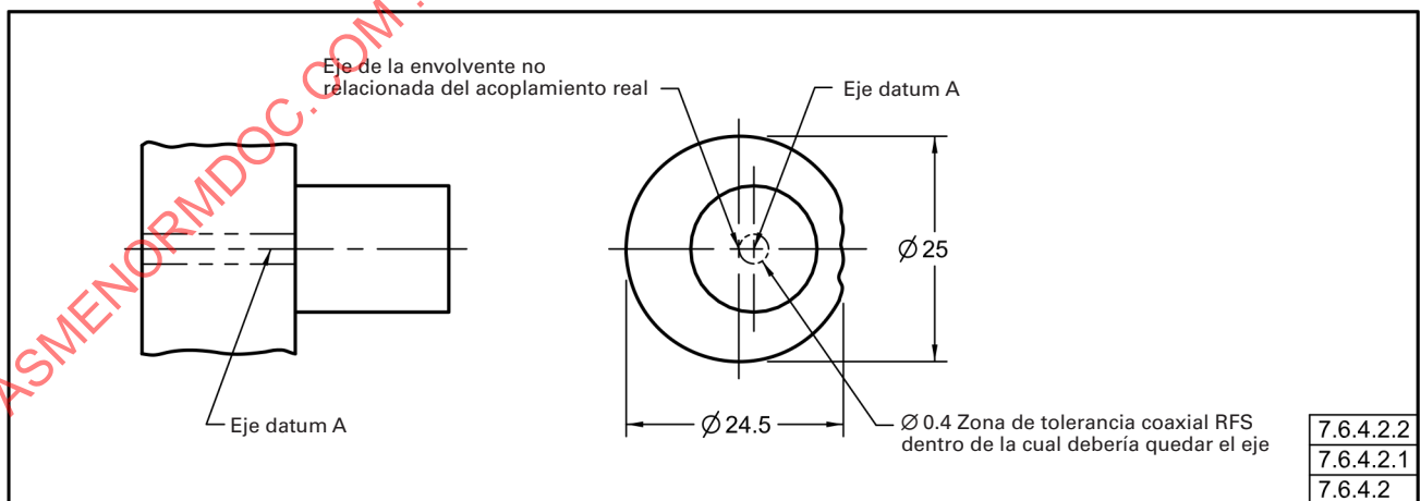
Fig. 7-61 Una Posible Configuración Aceptable de la Pieza Mostrada en la Fig. 7-57
