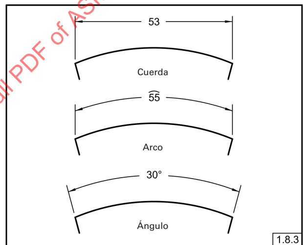
Fig. 1-28 Dimensionado de Cuerdas, Arcos y Ángulos
