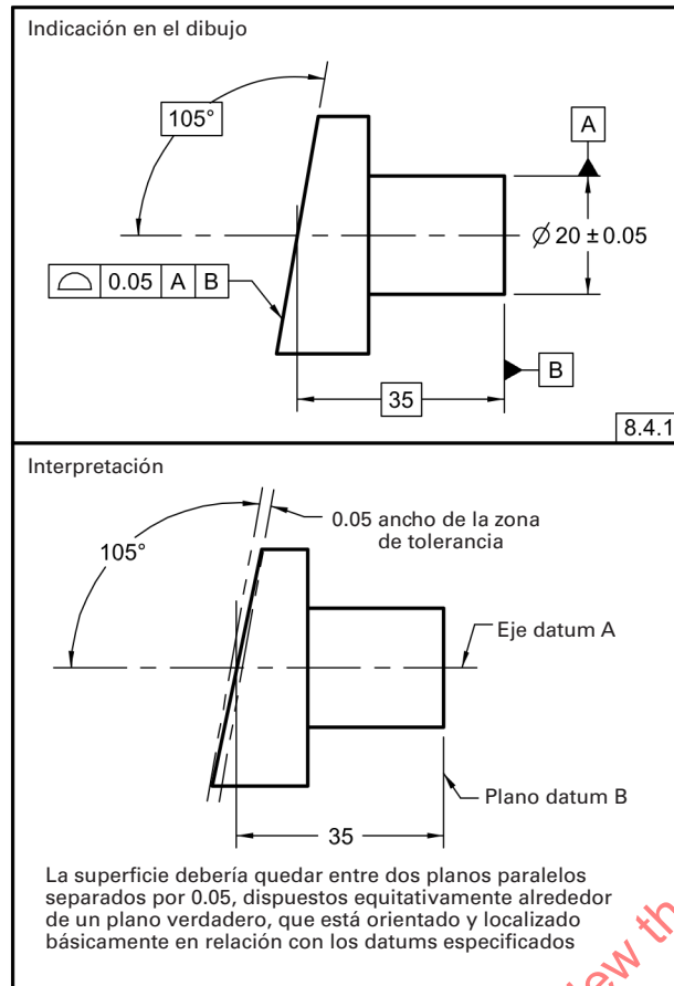
Fig. 8-13 Especificación del Perfil de una Superficie para una Superficie Plana
