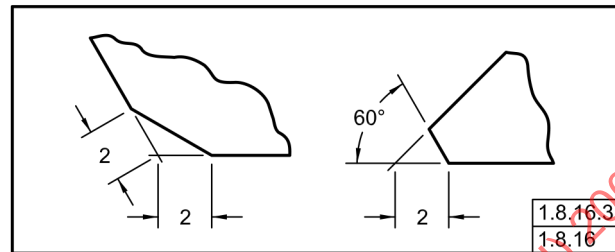
Fig. 1-45 Chaflanes entre Superficies Diferentes a 90°
