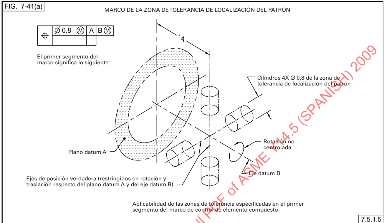
Fig. 7-41 Patrón Radial de Orificios Localizado por medio de Tolerancia Compuesta de Posición (Continuación) (Zonas de Tolerancia para Patrones Radiales de Orificios)
