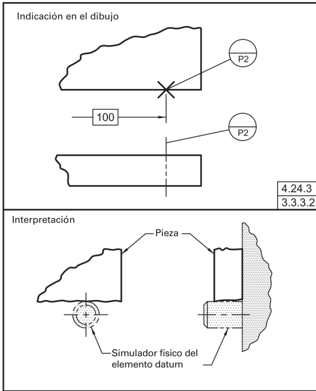
Fig 3-8 Datum objetivo de línea
