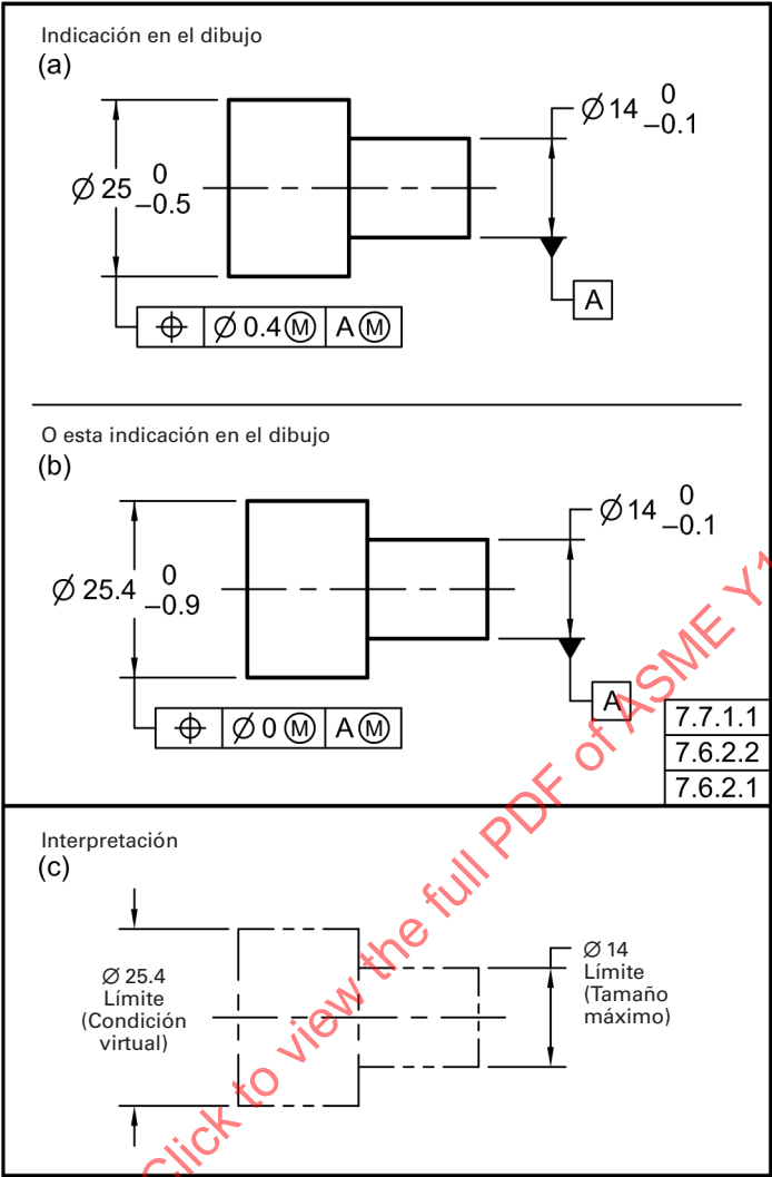
Fig. 7-56 Tolerancia de Posición para Coaxialidad
