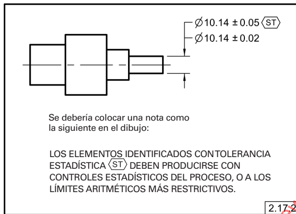
Fig. 2-25 Tolerancia Estadística con Límites Aritméticos
