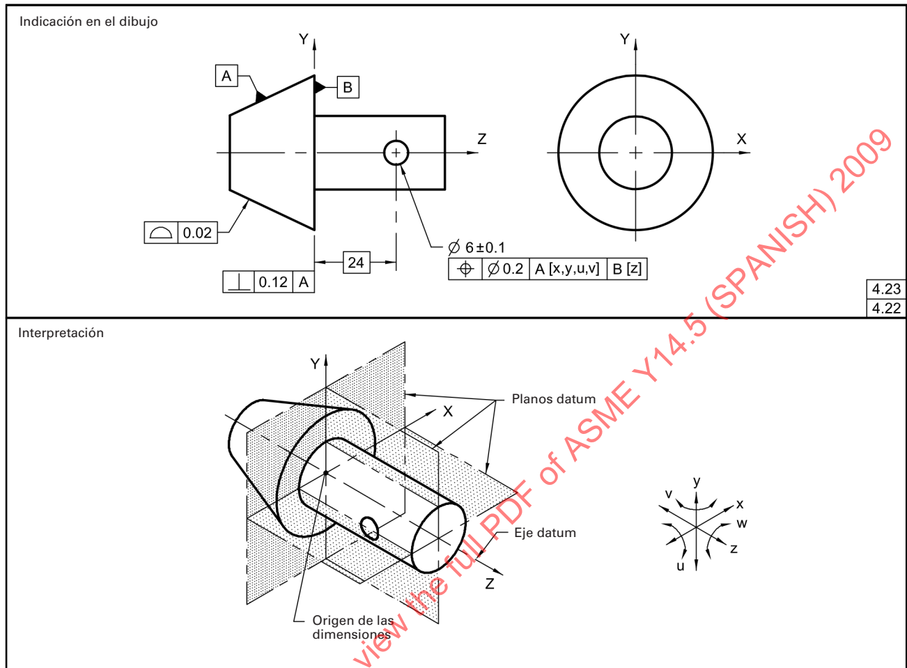
Fig. 4-45 Elemento Datum Cónico
