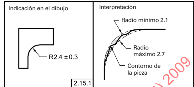
Fig. 2-22 Especificación de un Radio
