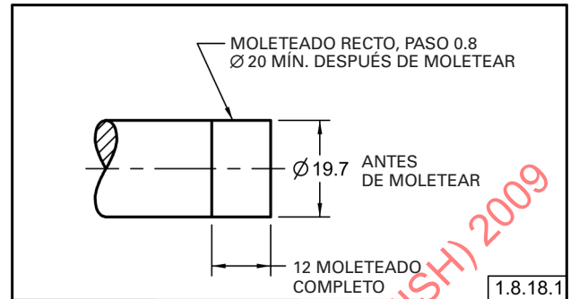
Fig. 1-48 Moleteados para ajustes a presión
