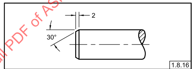
Fig. 1-42 Chaflanes
