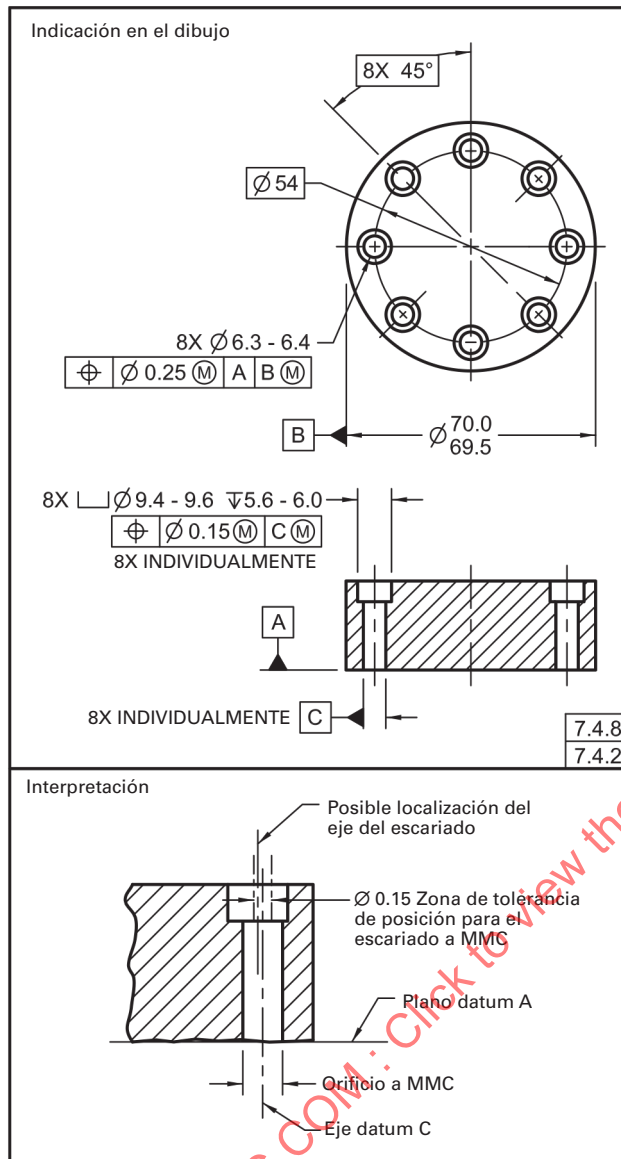
Fig. 7-26 Tolerancias de Posición para Orificios y Escariados, Diferentes Datums de Referencia
