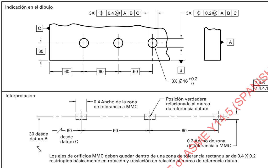
Fig. 7-28 Tolerancia de Posición Bidireccional, Método de Coordenadas Rectangulares
