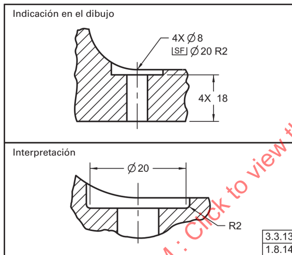
Fig. 1-41 Orificios refrentados
