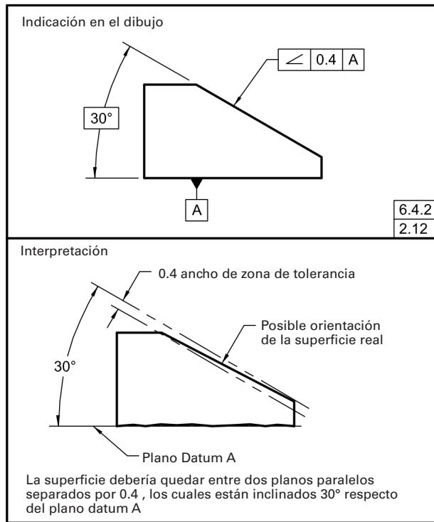
Fig. 6-1 Especificación de la Angularidad para una Superficie Plana
