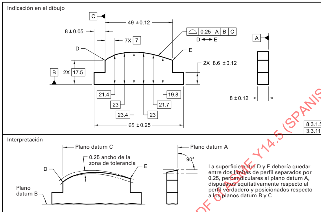
Fig. 8-7 Especificación del Perfil de una Superficie Entre Puntos
