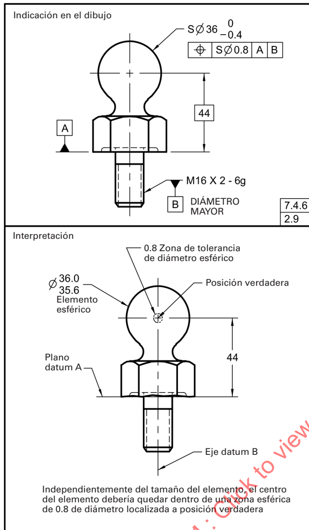
Fig. 7-35 Elemento Esférico Localizada por la Tolerancia de Posición
