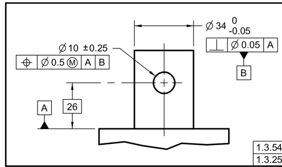
Fig. 1-1 Envolvere de Acoplamiento Real Relacionada y No Relacionada
