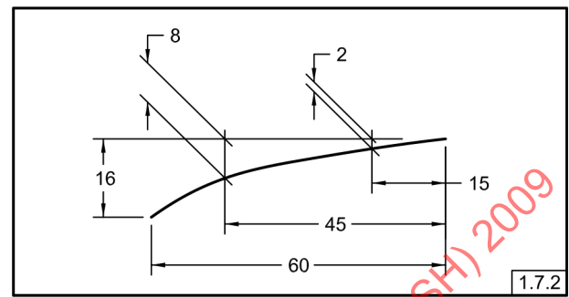
Fig. 1-10 Líneas de Extensión Oblicuas
