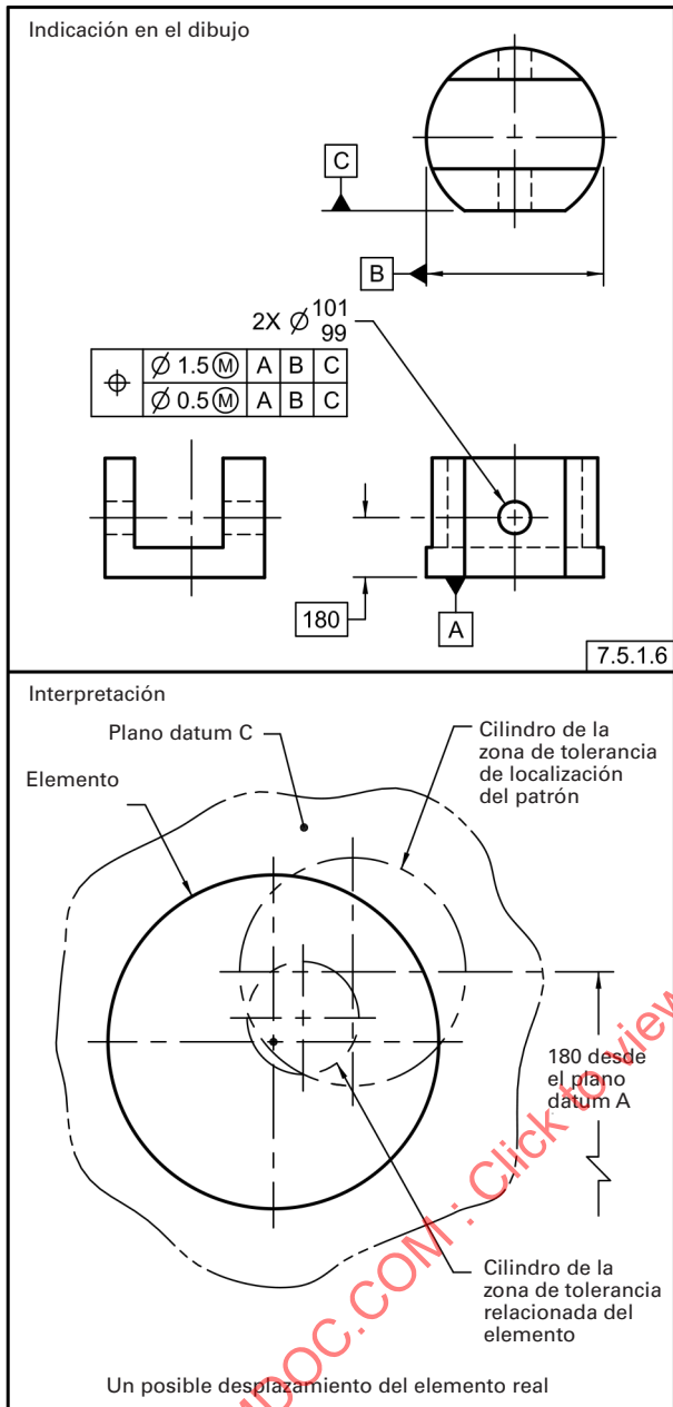
Fig. 7-43 Orientación Relativa a Tres Planos Datum
