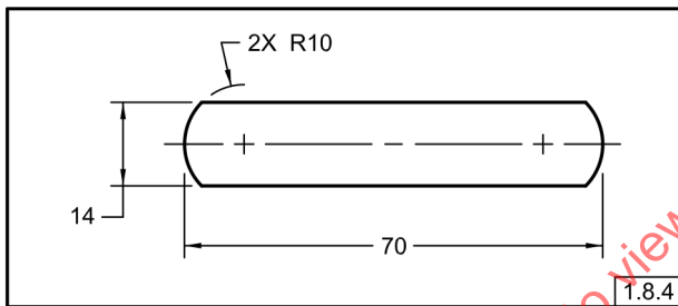
Fig. 1-30 Extremos Parcialmente Redondeados
