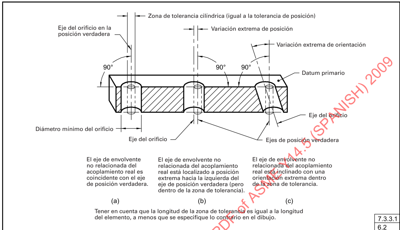
Fig. 7-8 Ejes de orificio en Relación con las Zonas de Tolerancia de Posición
