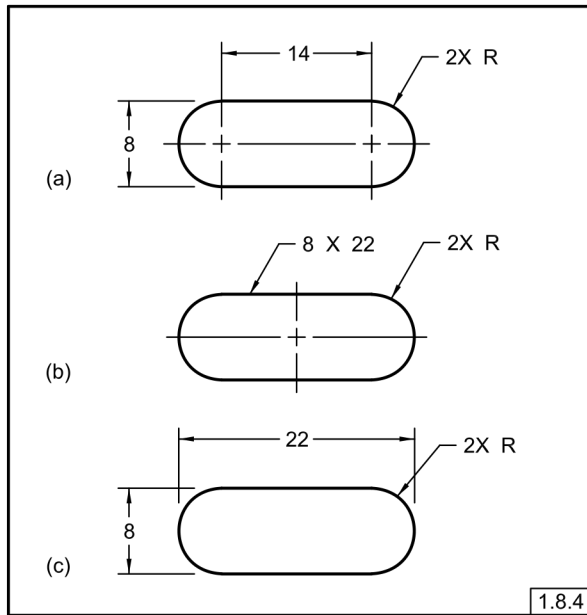
Fig. 1-29 Orificios Alargados
