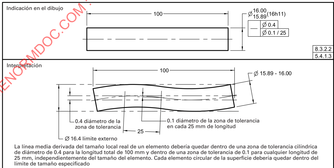
Fig. 5-4 Especificación de la Rectitud por Longitud de Unidad con Rectitud Total Especificada, Ambas en RFS
