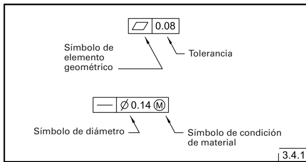
Fig. 3-23 Marco de Control del elemento
