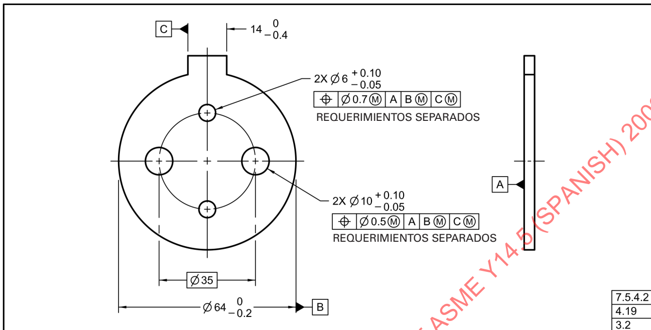
Fig. 7-54 Patrones Múltiples de Elementos, Requerimientos Separados
