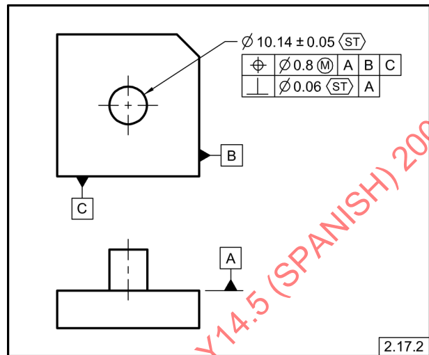
Fig. 2-26 Tolerancia Estadística con Controles Geométricos
