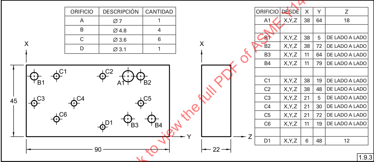
Fig. 1-51 Dimensionado por Coordenadas Rectangulares en Forma Tabular
