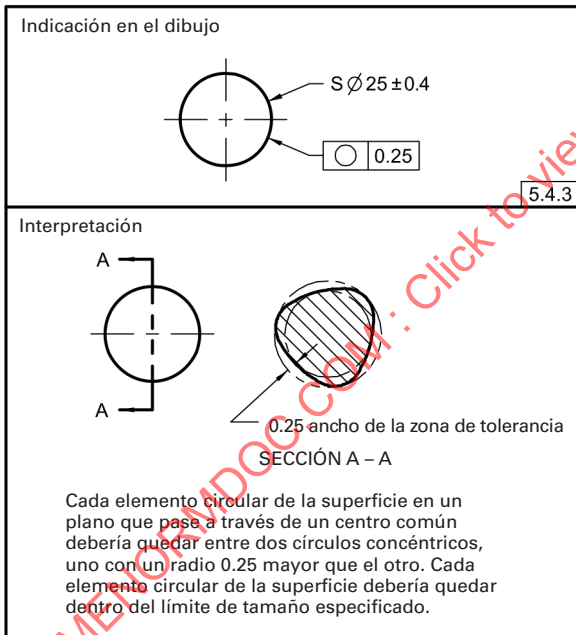
Fig. 5-11 Especificación de la Circularidad de una Esfera
