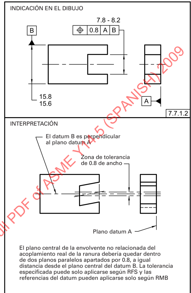
Fig. 7-65 Tolerancia de Posición RFS para Elementos Simétricos
