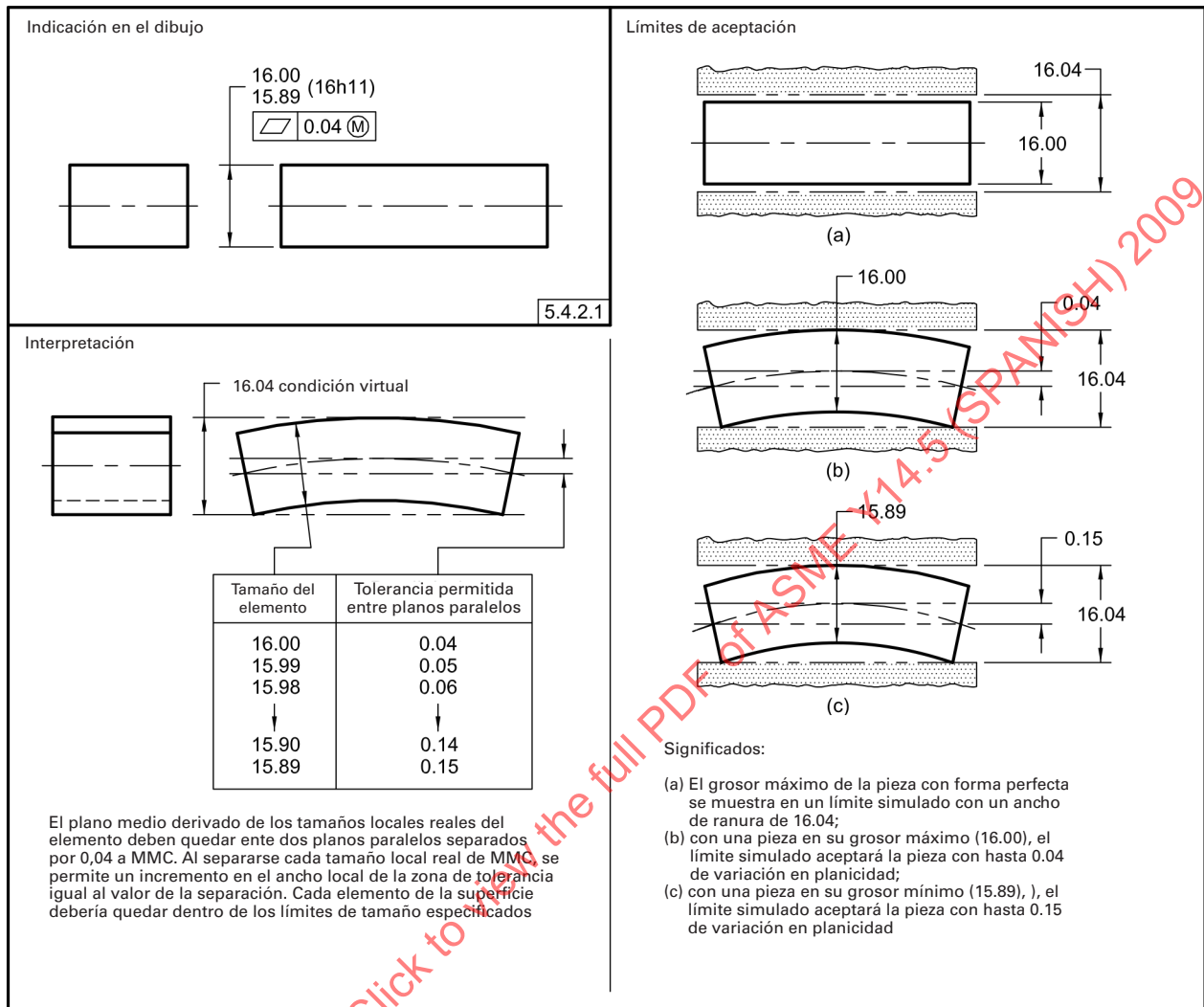
Fig. 5-9 Especificación de la Planicidad de un Plano Medio Derivado a MMC
