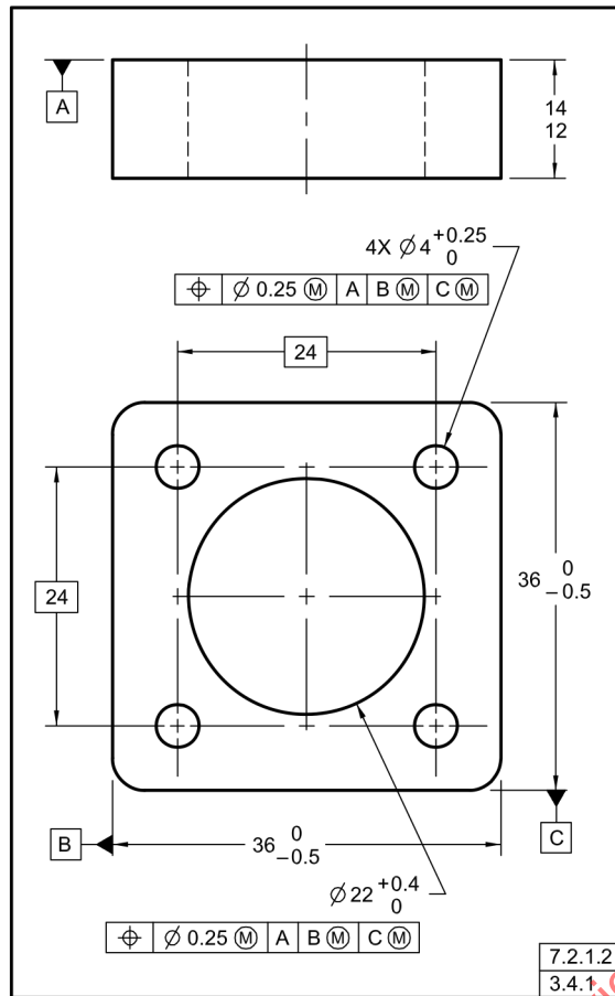
Fig. 7-4 Tolerancia de Posición a MMC en Relación con de Planos Centrales de Elementos Datum
