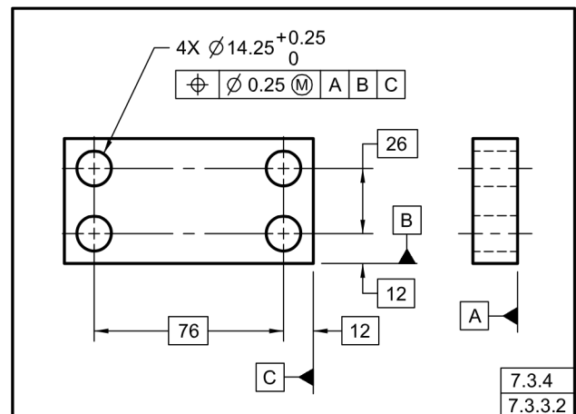
Fig. 7-10 Tolerancia de Posición a MMC
