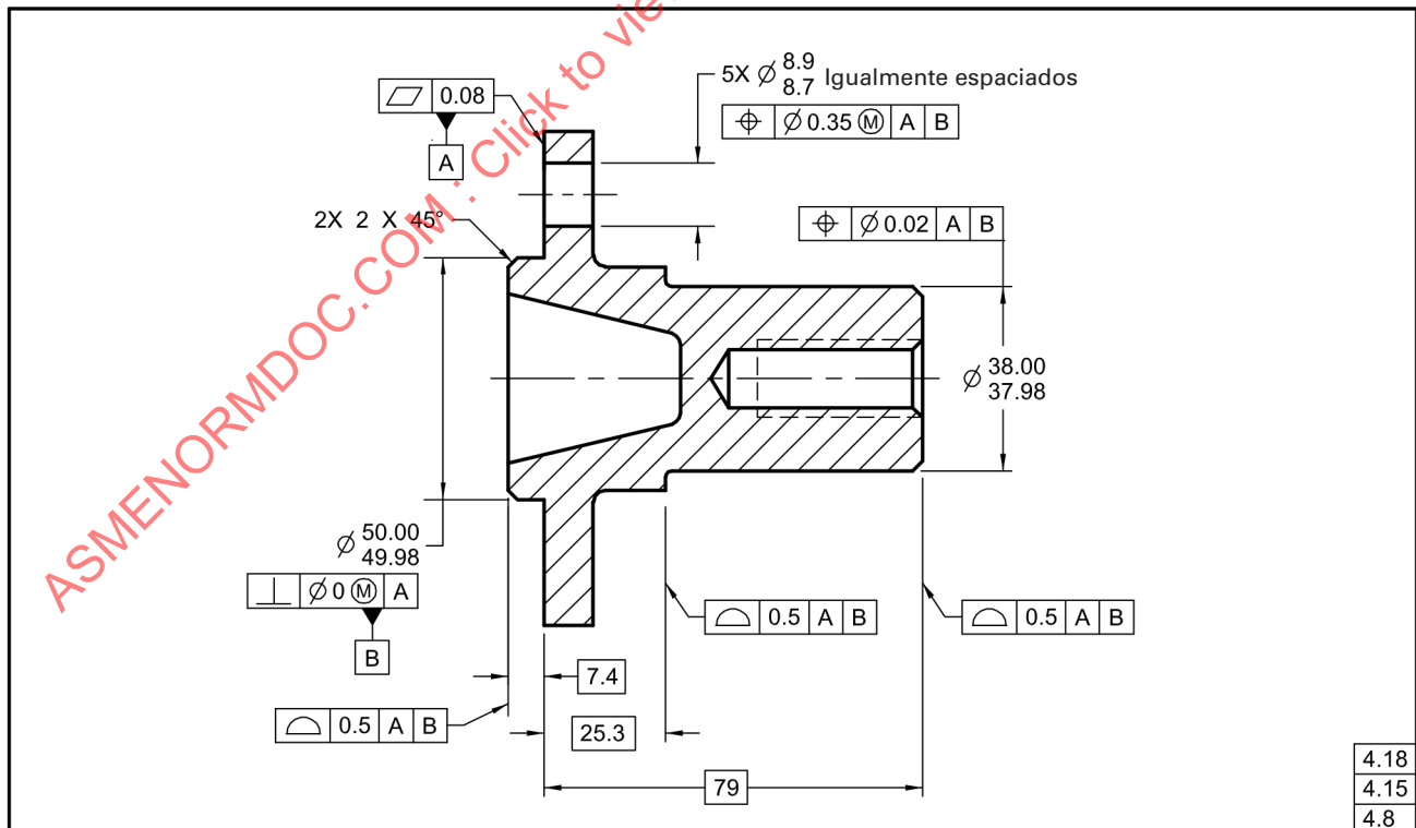
Fig. 4-38 Aplicación de Datum Funcional – Adaptador
