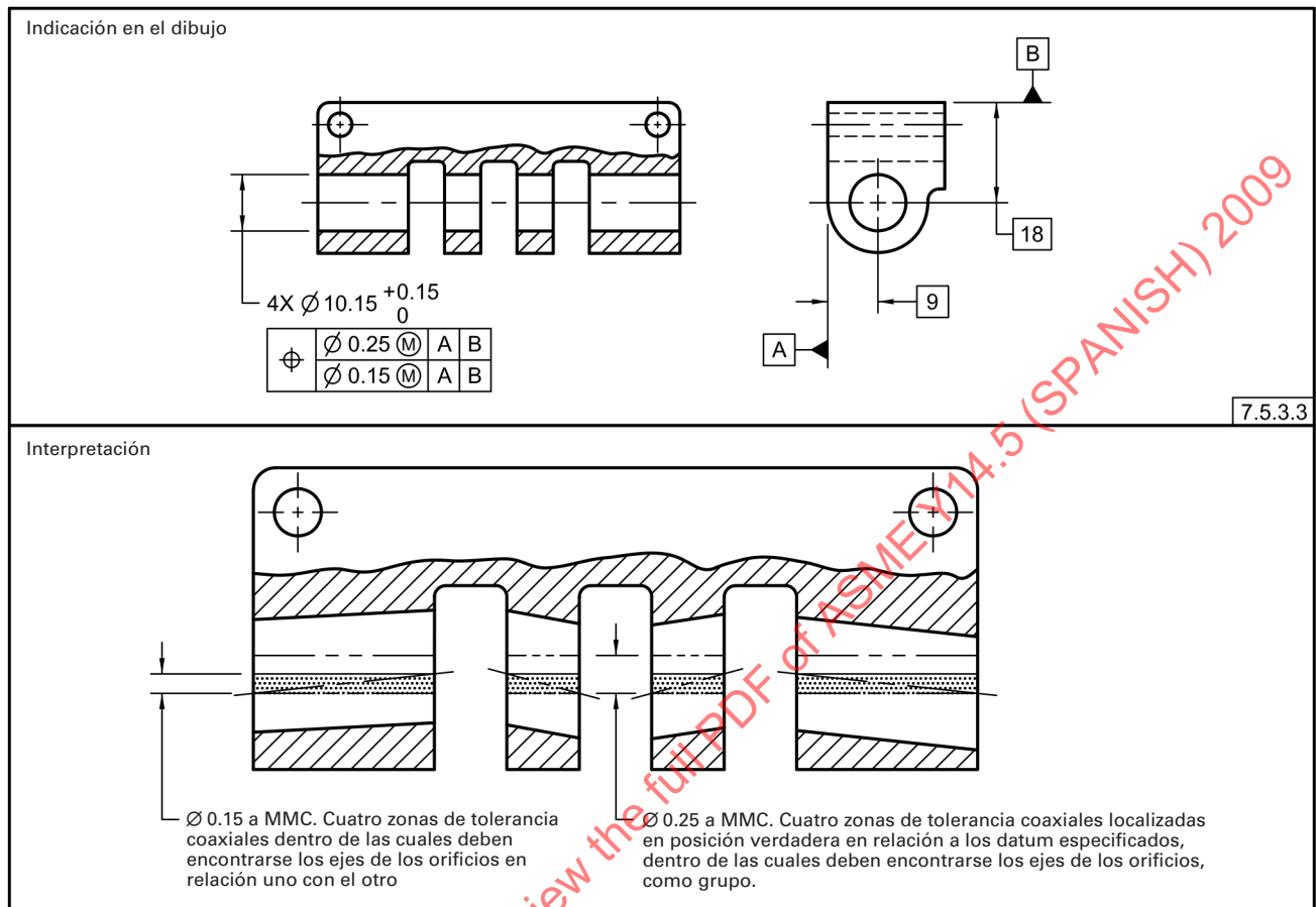
Fig. 7-50 Tolerancia de Posición para Orificios Coaxiales del Mismo Tamaño, Refinamiento Parcial (Paralelismo) del Eje Relacionado al Elemento.
