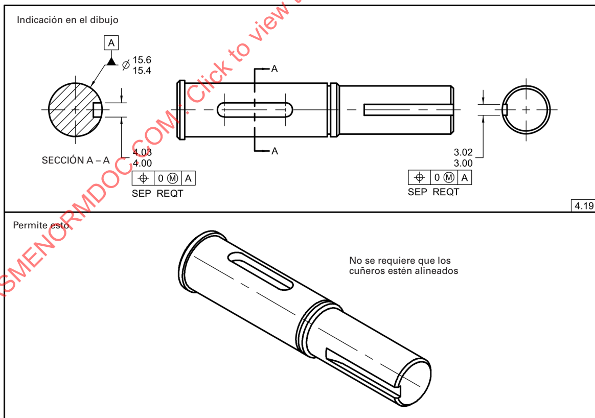
Fig. 4-41 Patrón de Elementos No Alineados – Requerimientos Separados Especificados
