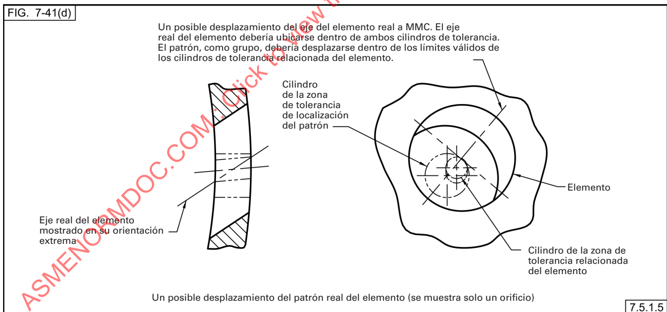
Fig. 7-41 Patrón Radial de Orificios Localizado por medio de Tolerancia Compuesta de Posición (Continuación) (Zonas de Tolerancia para Patrones Radiales de Orificios)
