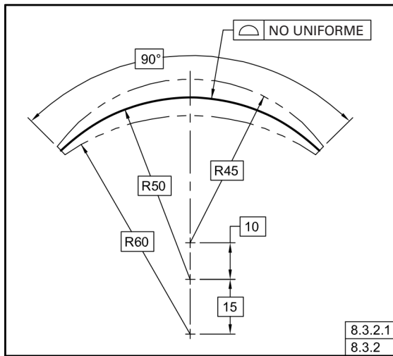
Fig. 8-9 Zona de Tolerancia No uniforme de Perfil
