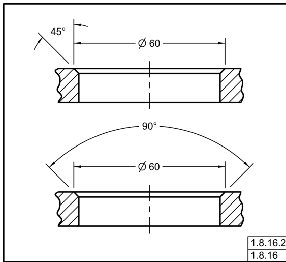
Fig. 1-44 Chaflanes Internos
