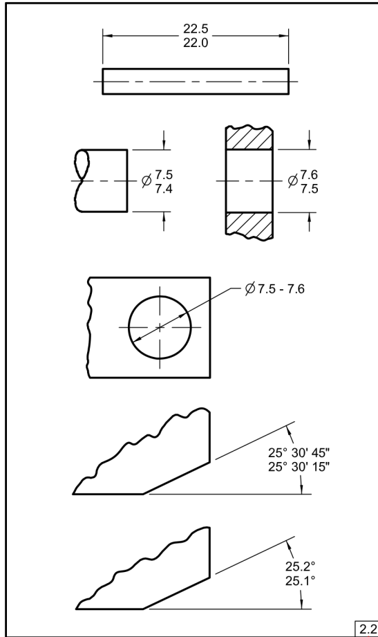
Fig. 2-1 Dimensionado por Límites
