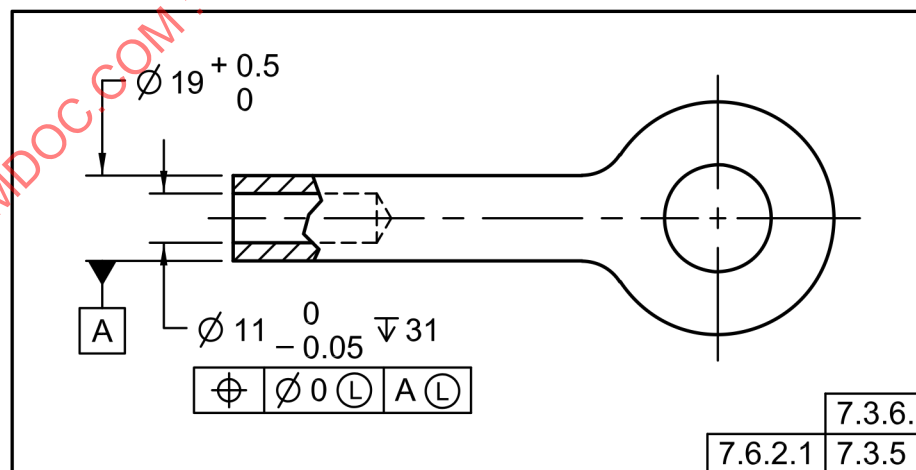
Fig. 7-17 Elemento Datum a LMB
