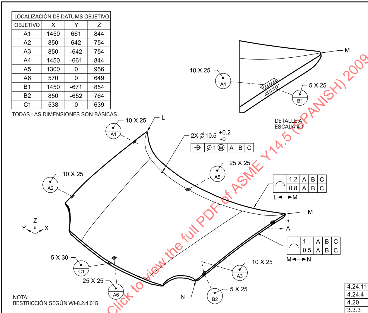
Fig. 4-42 Aplicación de Condición Restringida
