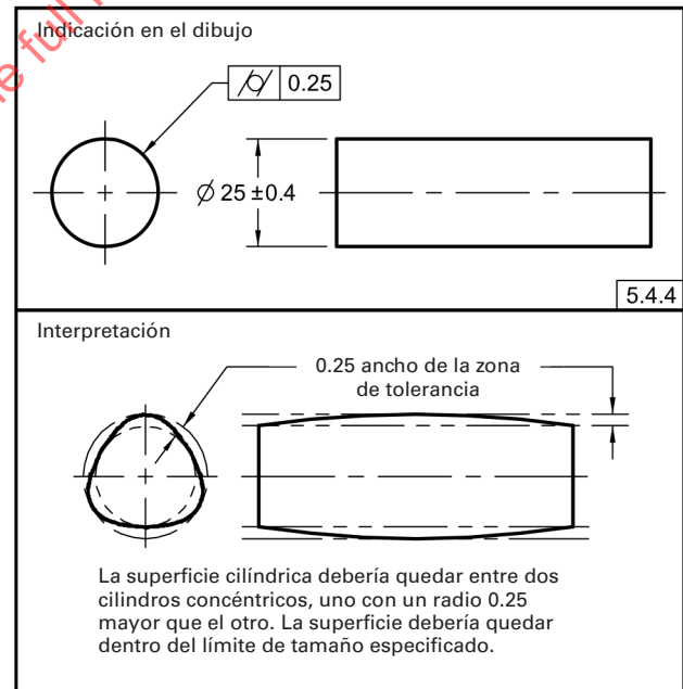
Fig. 5-12 Especificación de la Cilindricidad
