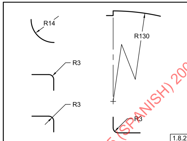
Fig. 1-22 Radios
