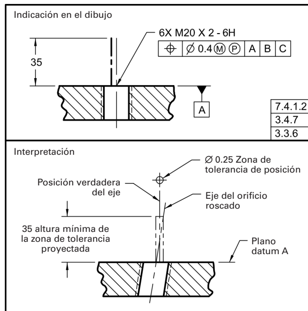
Fig. 7-22 Zona de Tolerancia Proyectada Indicada con Cadena
