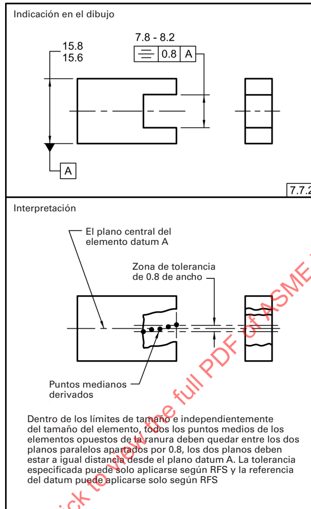
Fig. 7-66 Tolerancia de Simetría
