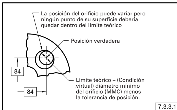
Fig. 7-7 Límite para la Superficie de un Orificio a MMC
