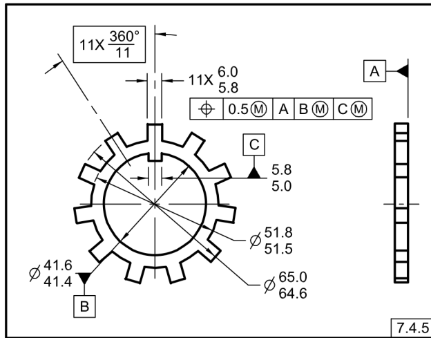
Fig. 7-30 Tolerancia de Posición de Pestañas
