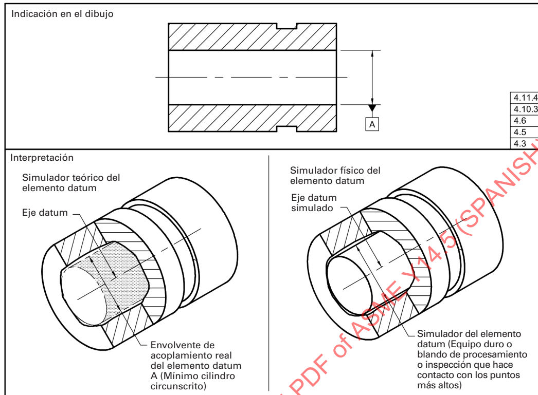
Fig. 4-12 Establecimiento de Datums – Para Elementos Cilíndricos Internos – RMB
