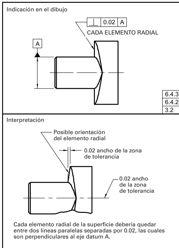
Fig. 6-16 Especificación de la Perpendicularidad para un Elemento Radial de una Superficie
