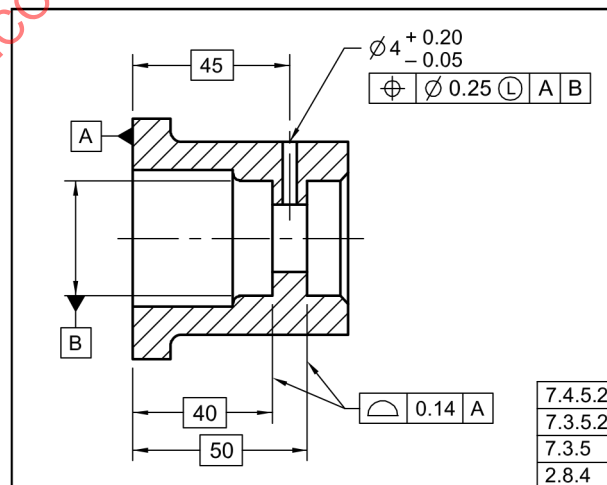
Fig. 7-15 LMC Aplicada a un Elemento Individual
