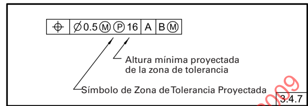
Fig. 3-28 Marco de Control del Elemento con un Símbolo de Zona de Tolerancia Proyectada
