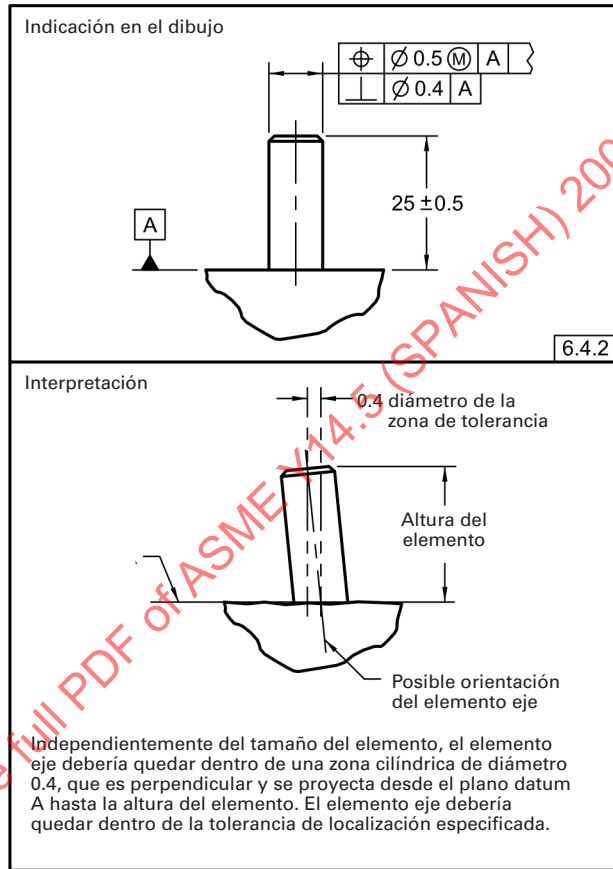
Fig. 6-12 Especificación de la Perpendicularidad para un Eje (Perno o Realce RFS)
