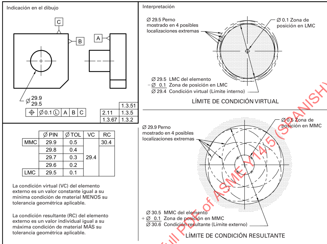
Fig. 2-16 Límites de Condición Virtual y Resultante Usando el Concepto LMC – Elemento Externo
