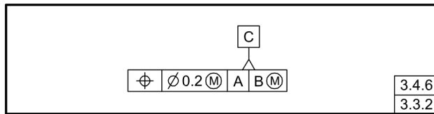
Fig. 3-27 Marco de Control de Elemento Combinado y Símbolo de Elemento Datum
