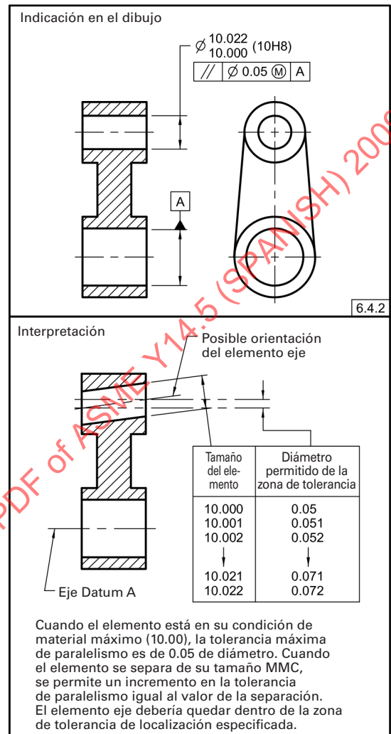
Fig. 6-10 Especificación del Paralelismo para un Eje (Elemento a MMC y Elemento Datum RFS)
