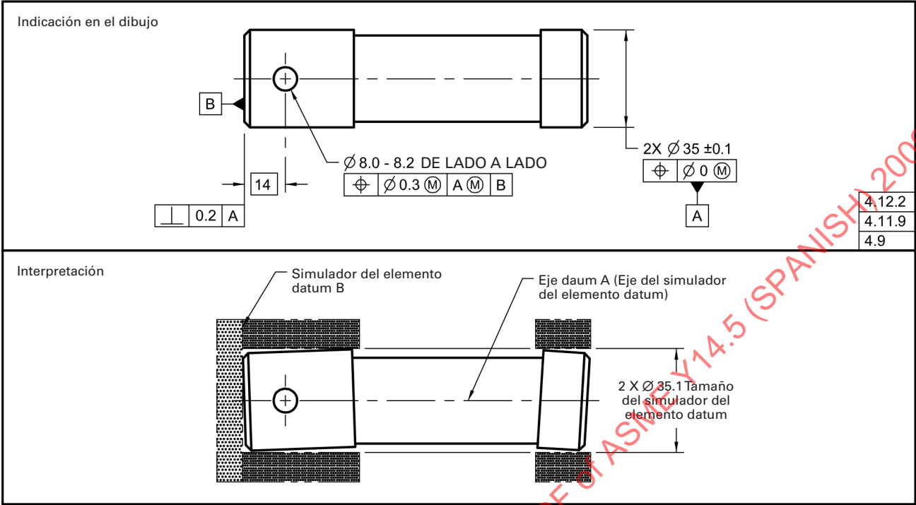
Fig. 4-24 Dos Elementos Datum Coaxiales, Eje Datum Individual
