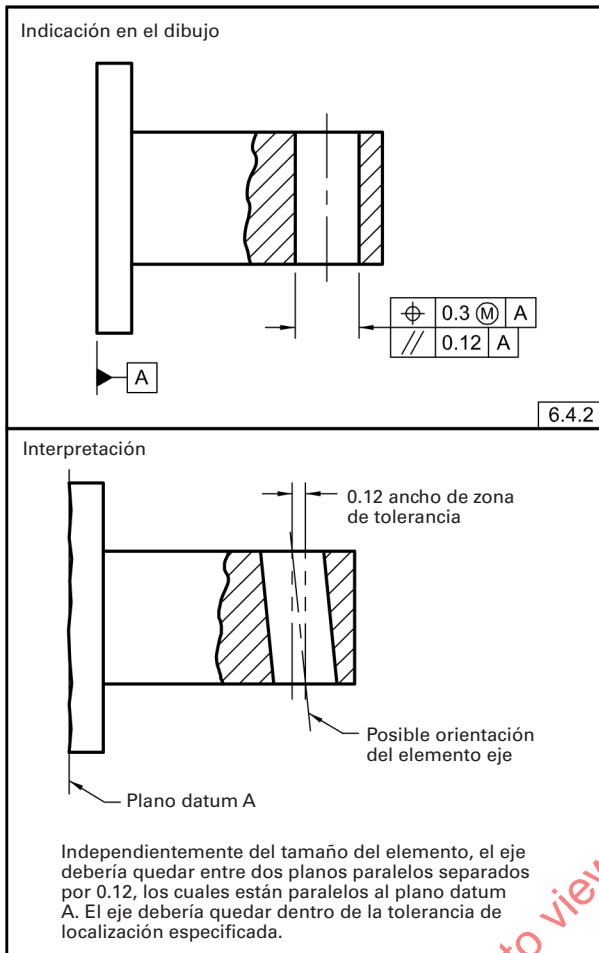
Fig. 6-7 Especificación del Paralelismo para un Eje (Elemento RFS)
