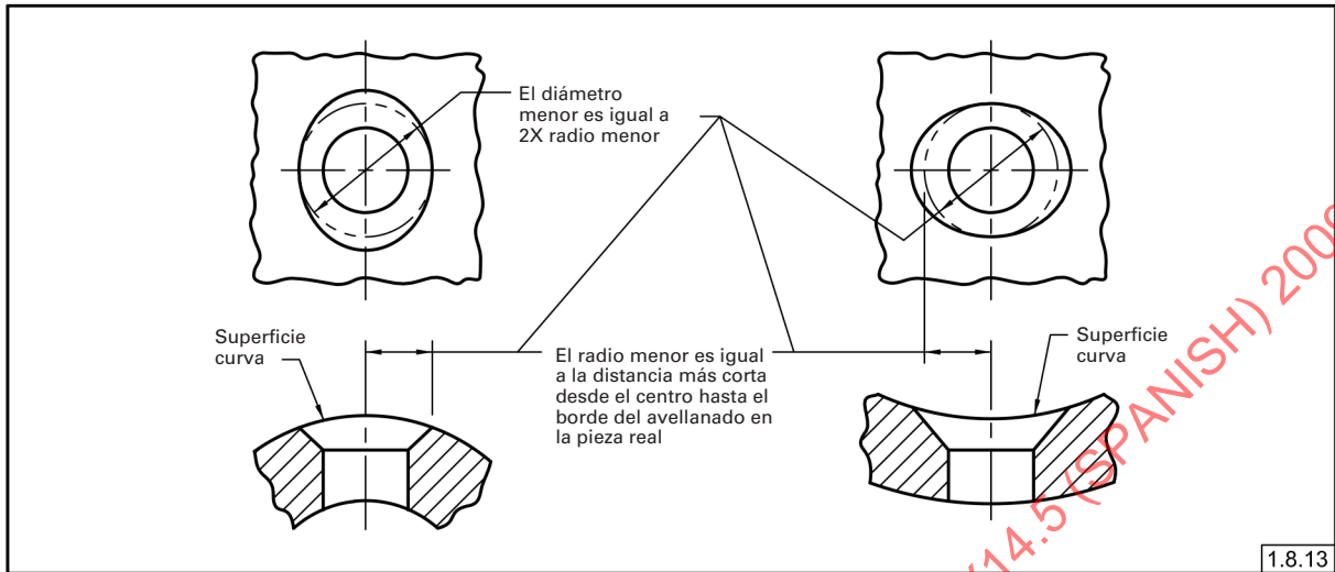
Fig. 1-40 Avellanado en una superficie curva
