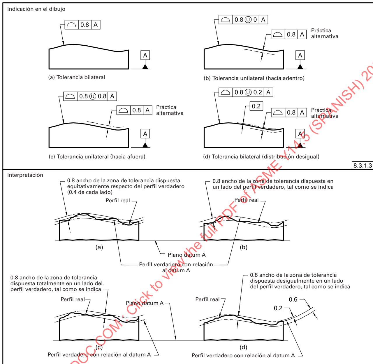
Fig. 8-4 Aplicación de la Tolerancia de un Perfil de Superficie Respecto a un Contorno Básico
