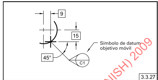
Fig. 3-22 Aplicación del Símbolo de Datum Objetivo Móvil
