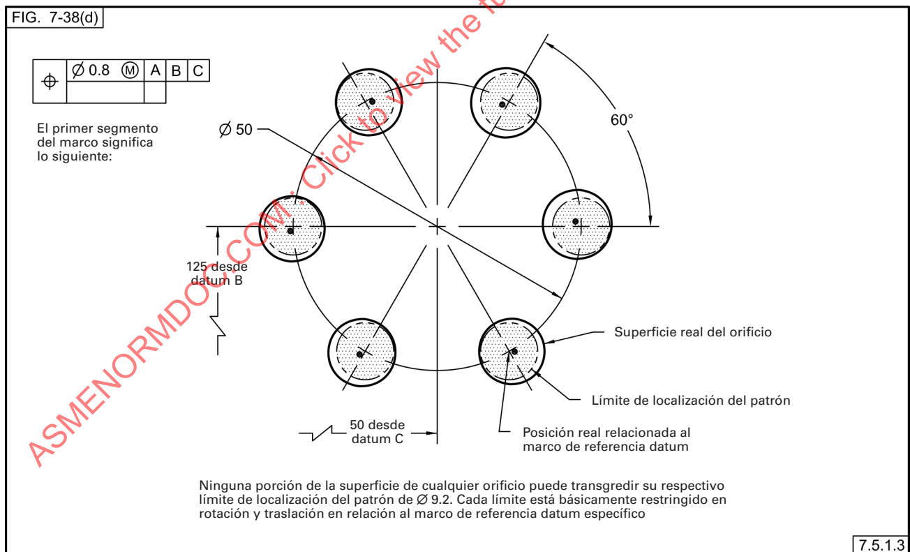
Fig. 7-38 Patrón de Orificios Localizados por Tolerancia Compuesta de Posición (Continuación) (Zonas de Tolerancia para Patrón de Orificios)
