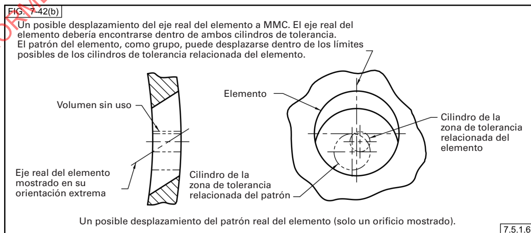
Fig. 7-42 Patrón Radial de Orificios Localizado por medio de Tolerancia Compuesta de Posición (Continuación) (Zonas de Tolerancia para Patrón Radial de Orificios)
