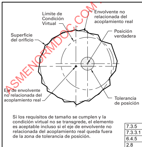
Fig. 7-6 Ilustración de la Diferencia Entre las Interpretaciones de Superficie y Eje de una Tolerancia de Posición para un Orificio Cilíndrico
