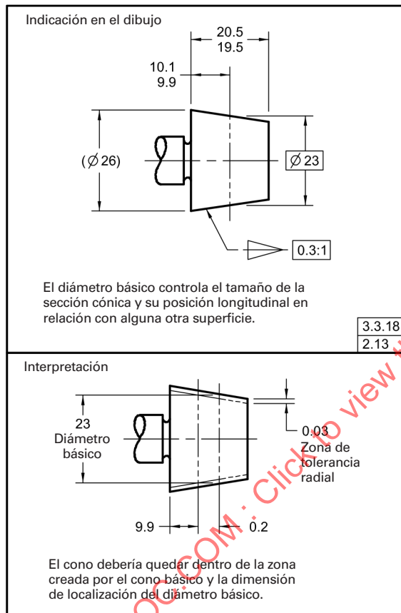
Fig. 2-21 Especificación de un Cono Básico y un Diámetro Básico
