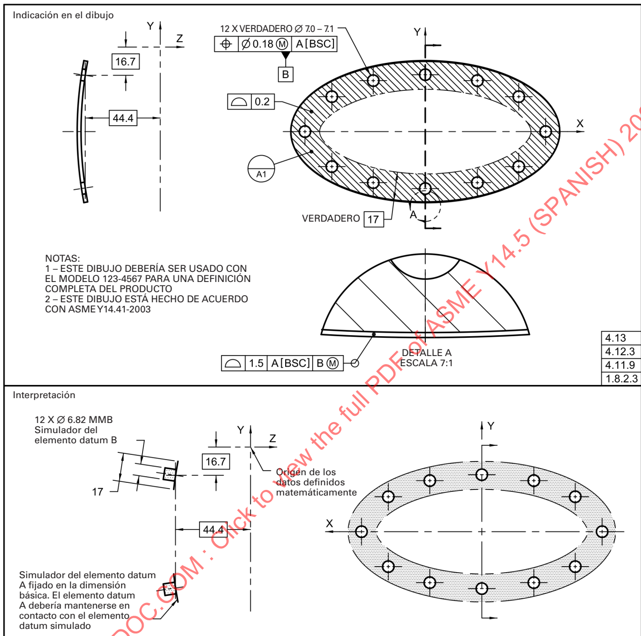
Fig. 4-28 Superficie de Contorno como un Elemento Datum
