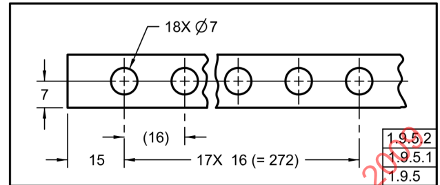
Fig. 1-55 Elementos y Dimensiones Repetitivos
