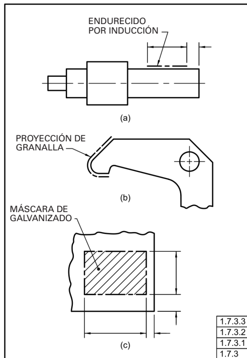
Fig. 1-13 Indicación de Longitud o Área Limitada
