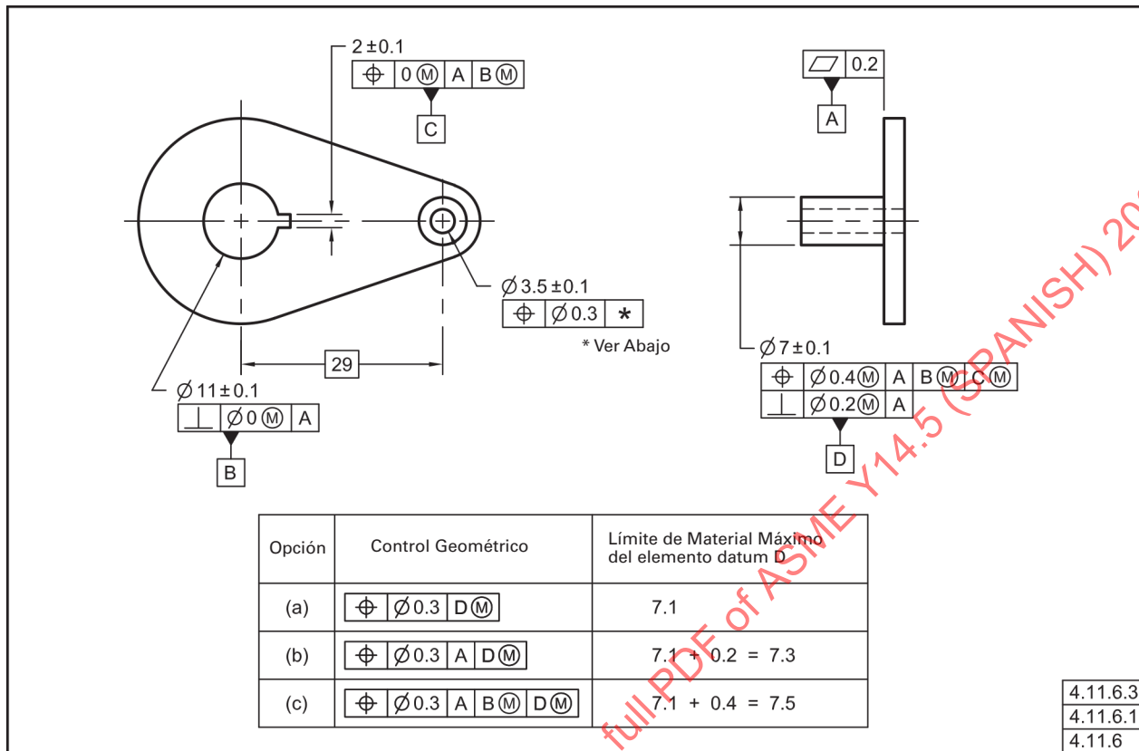
Fig. 4-16 Ejemplo de Cálculos del Límite de Material Máximo
