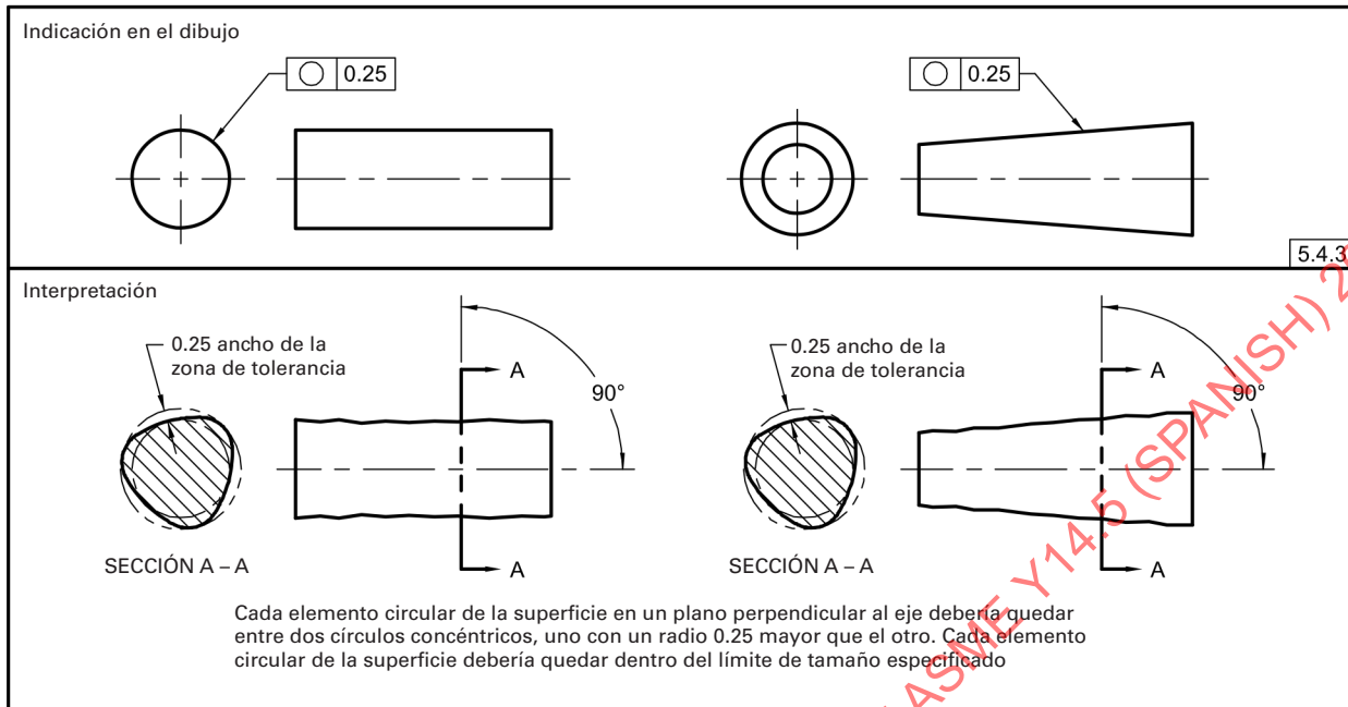
Fig. 5-10 Especificación de la Circularidad para un Cilindro o Cono
