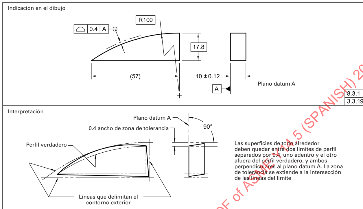
Fig. 8-12 Especificación del Perfil de una Superficie para Esquinas Agudas
