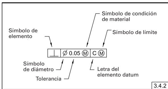
Fig. 3-24 Marco de Control de elemento con elemento datum de referencia
