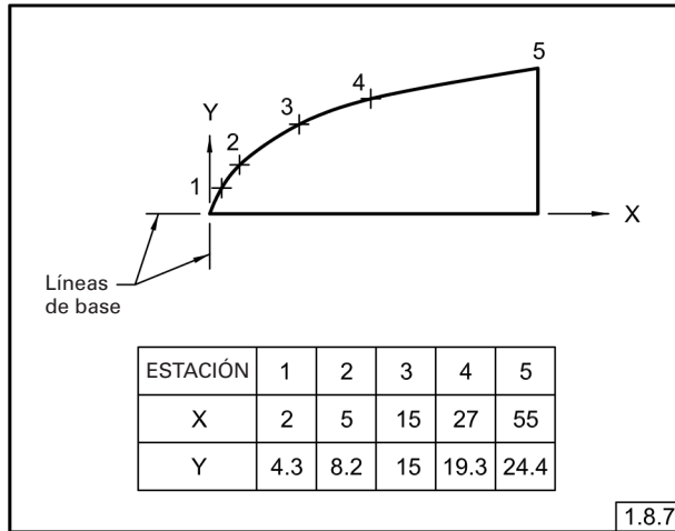
Fig. 1-34 Contorno Tabulado
