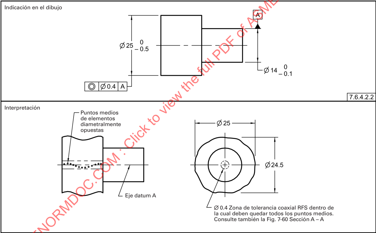
Fig. 7-63 Artículo Mostrado en la Fig. 7-57 Controlado para Concentricidad
