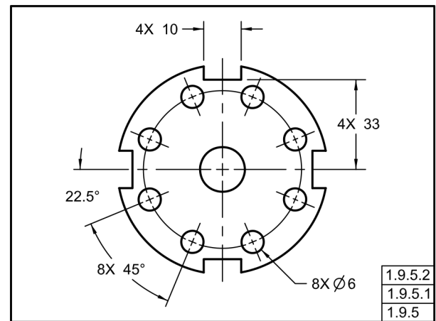
Fig. 1-57 Elementos y Dimensiones Repetitivos
