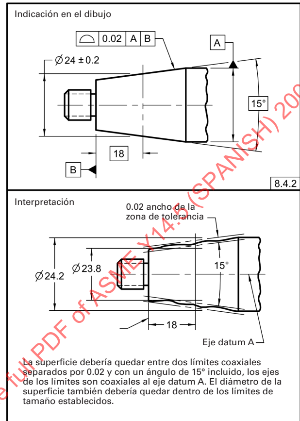
Fig. 8-18 Tolerancia de Perfil de un Elemento Cónico con Relación a Datums
