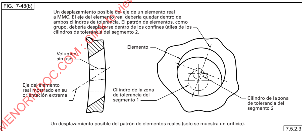
Fig. 7-48 Patrón Radial de Orificios Localizado por Marcos de Control de Elemento de Múltiples Segmentos Individuales (Continuación) (Zonas de Tolerancia para Patrón Radial de Orificios)
