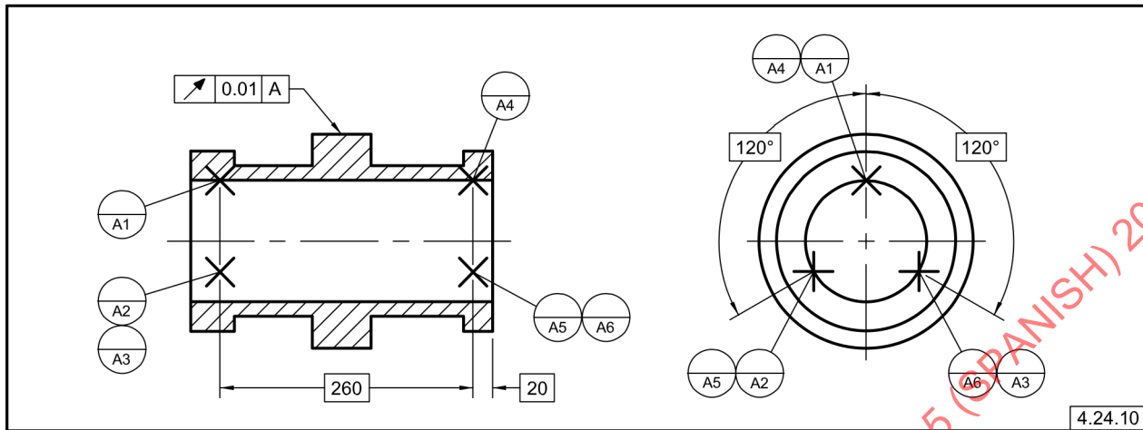
Fig. 4-50 Eje Datum Primario Establecido por Tres Puntos Datum Objetivo en un Elemento Cilíndrico Individual
