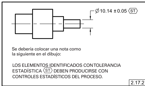
Fig. 2-24 Tolerancia Estadística
