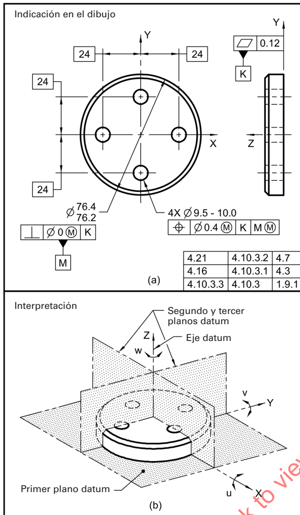
Fig. 4-8 Pieza con Elemento Datum Cilindrico
