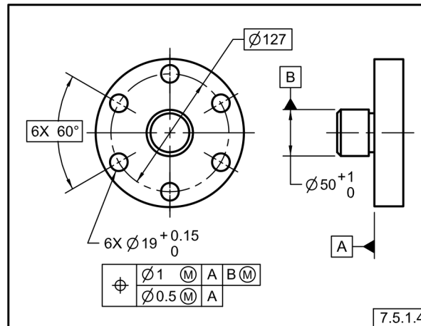
Fig. 7-40 Tolerancia Compuesta de Posición de un Patrón Circular de Elementos
