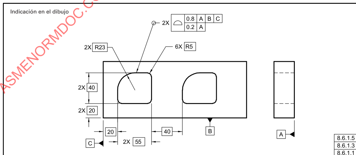
Fig. 8-21 Patrón Localizado por una Tolerancia de Perfil Compuesto
