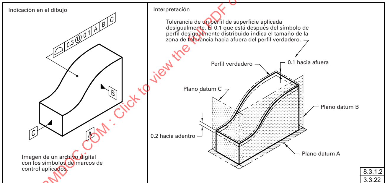
Fig. 8-3 Aplicación 3D de un Perfil de Superficie (Desigualmente Distribuida)
