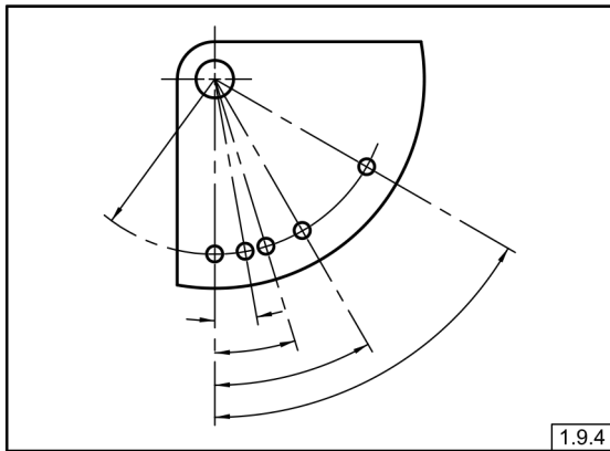
Fig. 1-52 Dimensionado con Coordenadas Polares
