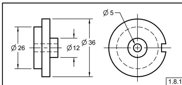
Fig. 1-21 Diámetros
