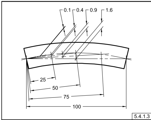
Fig. 5-5 Posibles Resultados de la Rectitud Especificada por Longitud de Unidad RFS, sin Especificar la Rectitud Total
