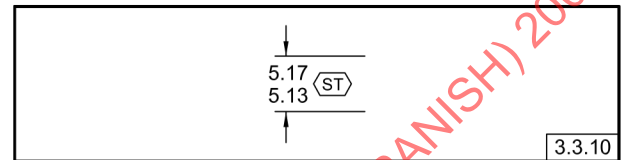
Fig. 3-13 Símbolo de Tolerancia Estadística
