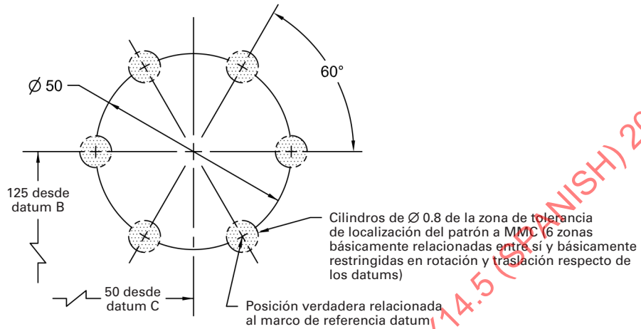
Fig. 7-38 Patrón de Orificios Localizados por Tolerancia Compuesta de Posición (Continuación) (Marco de la Zona de Tolerancia de Localización del Patrón – PLTZF)
