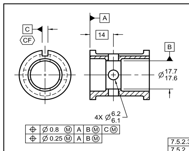
Fig. 7-48 Patrón Radial de Orificios Localizado por Marcos de Control de Elemento de Múltiples Segmentos Individuales
