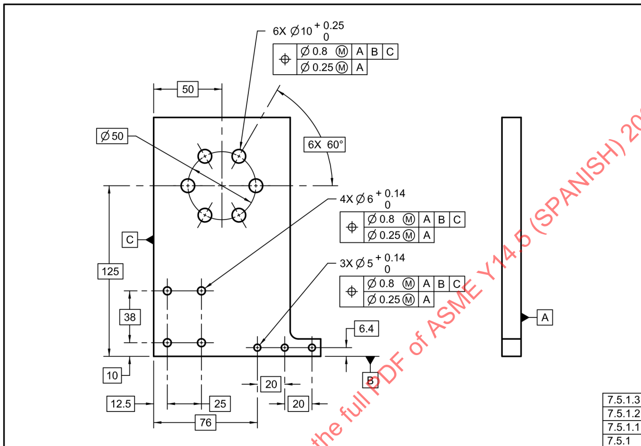
Fig. 7-38 Patrón de Orificios Localizados por Tolerancia Compuesta de Posición
