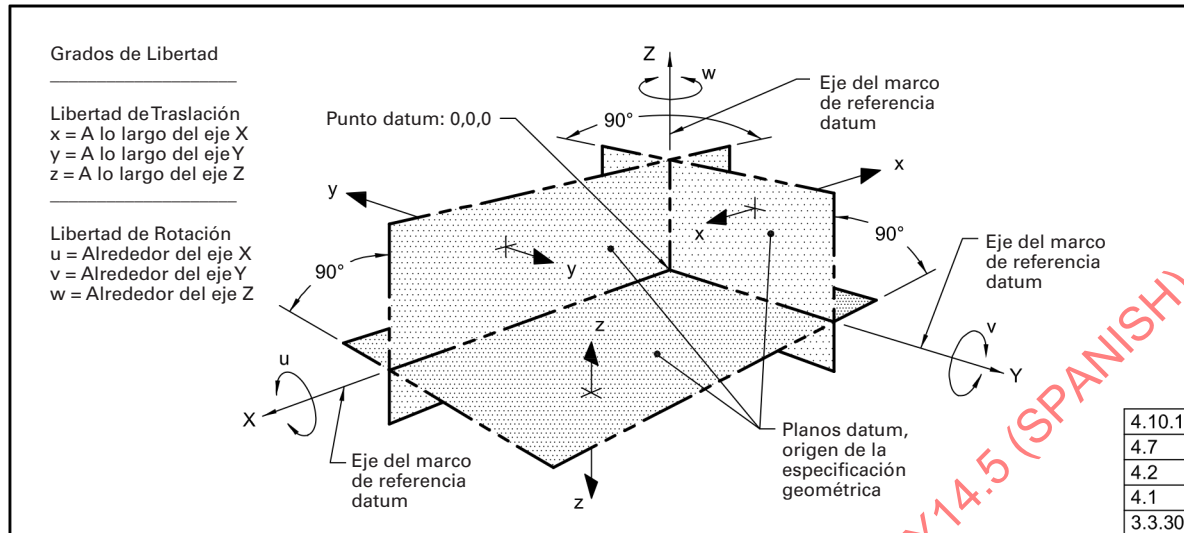
Fig. 4-1 Marco de Referencia Datum
