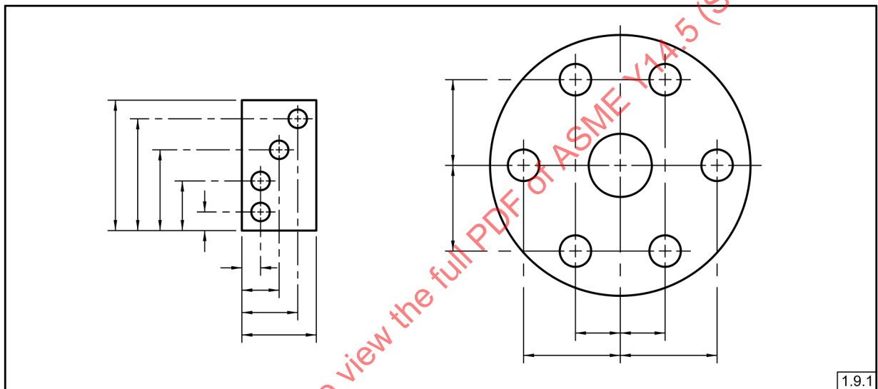
Fig. 1-49 Dimensionado con Coordenadas Rectangulares
