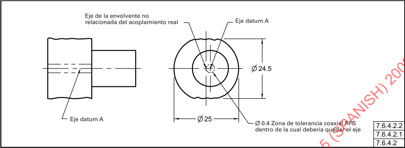
Fig. 7-62 Una Posible Configuración Aceptable de la Pieza Mostrada en la Fig. 7-57
