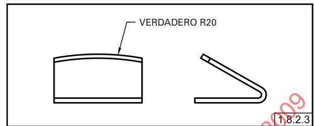
Fig. 1-26 Radio Verdadero
