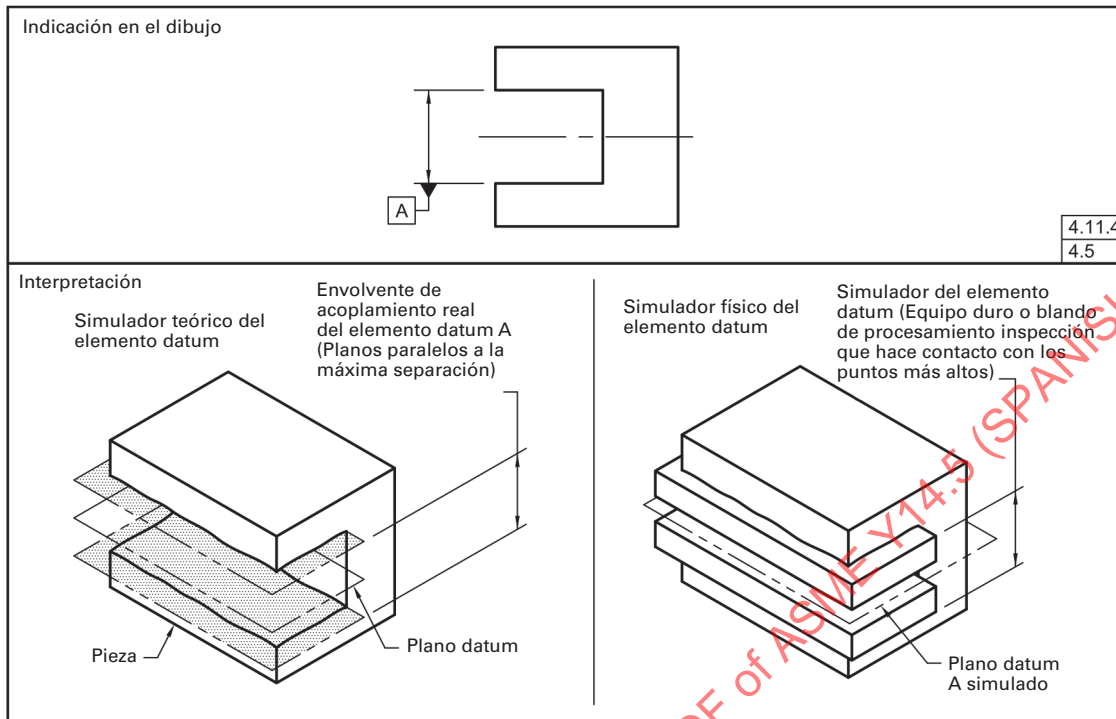
Fig. 4-14 Establecimiento de Datums – Para Ancho de Datum Interno – RMB
