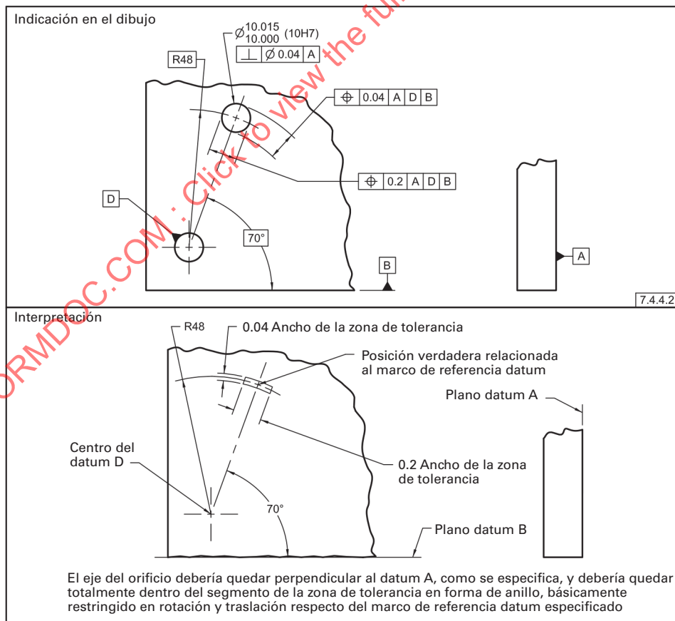
Fig. 7-29 Tolerancia de Posición Bidireccional, Método de Coordenadas Polares
