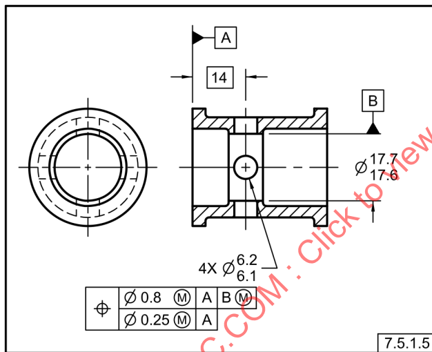
Fig. 7-41 Patrón Radial de Orificios Localizado por medio de Tolerancia Compuesta de Posición
