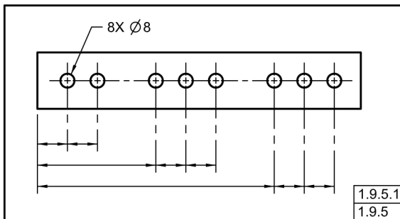
Fig. 1-53 Elementos Repetitivos
