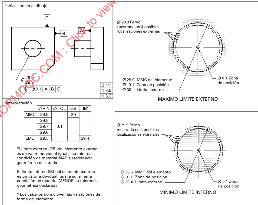
Fig. 2-17 Límites de Condición Internos y Externos Usando el Concepto RFS – Elemento Externo
