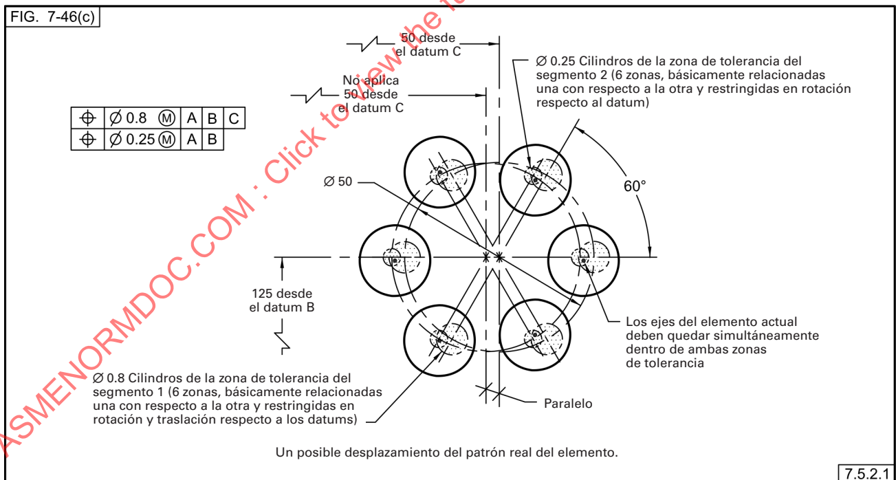
Fig. 7-46 Patrones de Orificios de la Fig. 7-46. Marcos de Control de Elemento de Múltiples Segmentos Individuales con Datum Secundario en el Marco de Control de Elemento Inferior (Continuación) (Zonas de Tolerancia para Patrón de Seis Orificios)
