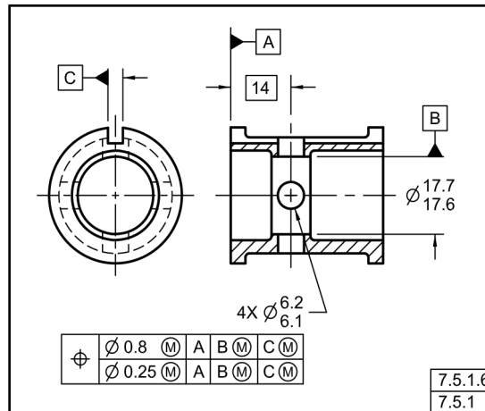
Fig. 7-42 Patrón Radial de Orificios Localizado por medio de Tolerancia Compuesta de Posición
