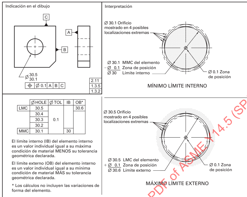
Fig. 2-14 Límites Internos y Externos Usando el Concepto RFS – Elemento Interno
