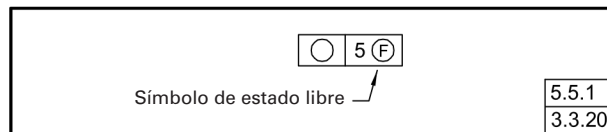
Fig. 3-21 Marco de Control del Elemento con el Símbolo de Estado Libre
