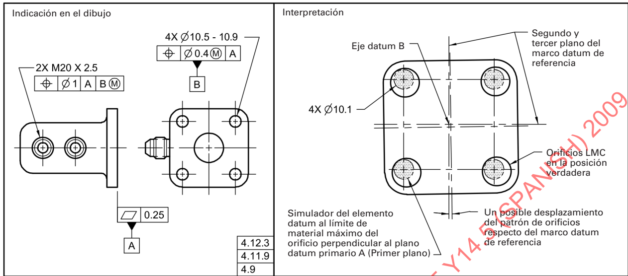
Fig. 4-26 Patrón de orificios Identificados como Datum
