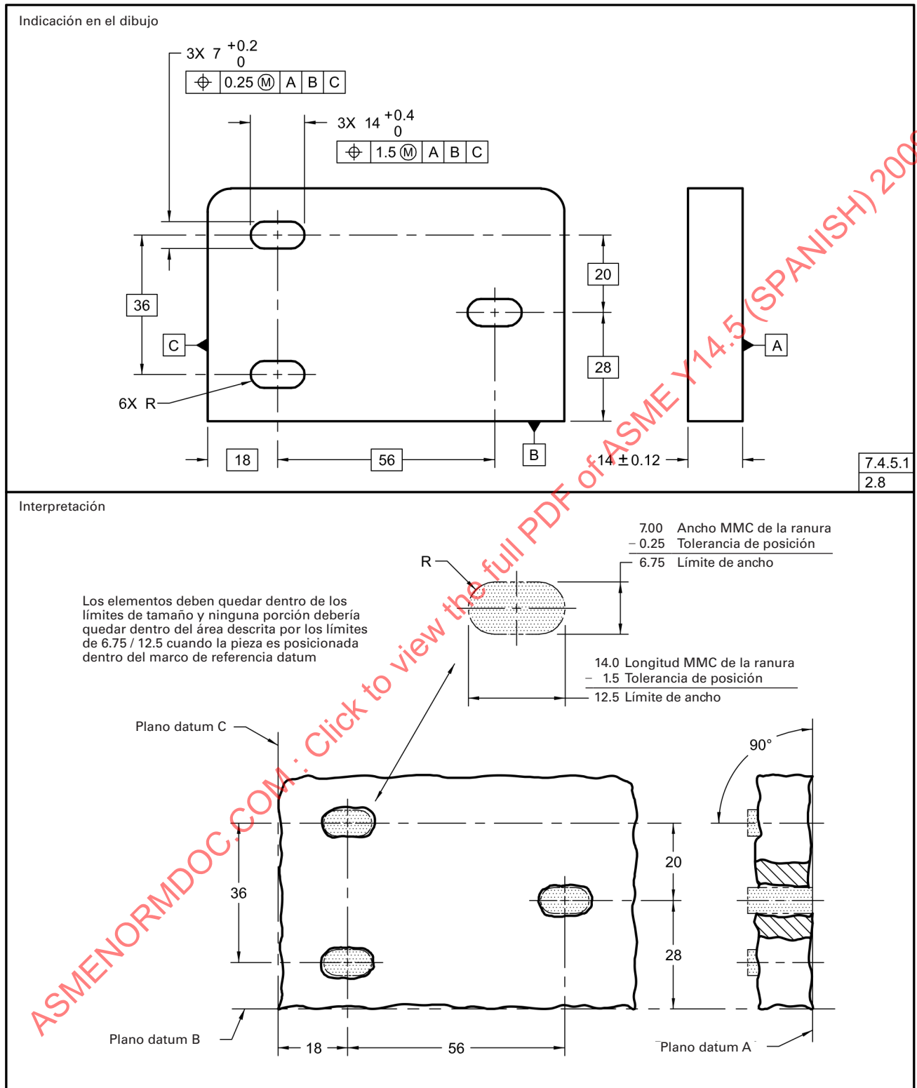
Fig. 7-34 Tolerancia de Posición, Concepto de Límites
