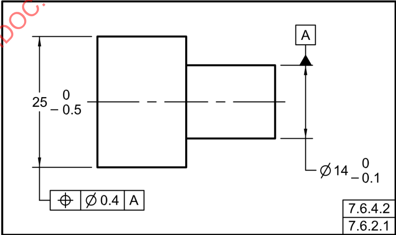
Fig. 7-57 Elemento Controlado con Tolerancia de Posición a RFS y Datum Referenciado a RMB para Coaxialidad
