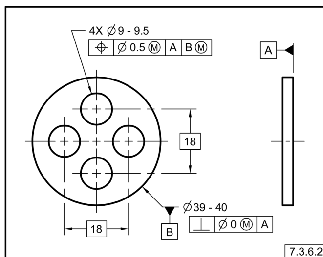
Fig. 7-18 Elemento Datum Referenciado a MMB
