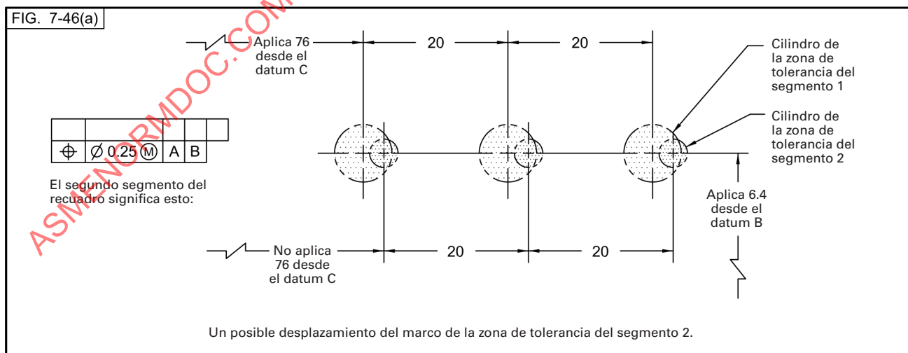
Fig. 7-46 Patrones de Orificios de la Fig. 7-46. Marcos de Control de Elemento de Múltiples Segmentos Individuales con Datum Secundario en el Marco de Control de Elemento Inferior (Continuación) (Zonas de Tolerancia para Patrón de Tres Orificios)
