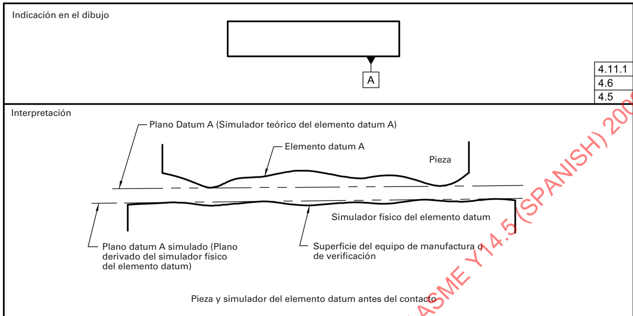
Fig. 4-10 Establecimiento del Plano Datum
