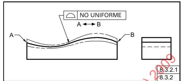
Fig. 8-10 Zona de Tolerancia No uniforme de Perfil
