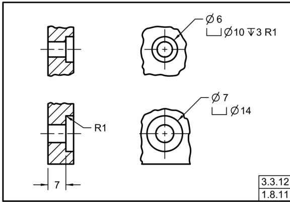
Fig. 1-37 Orificios Escariados
