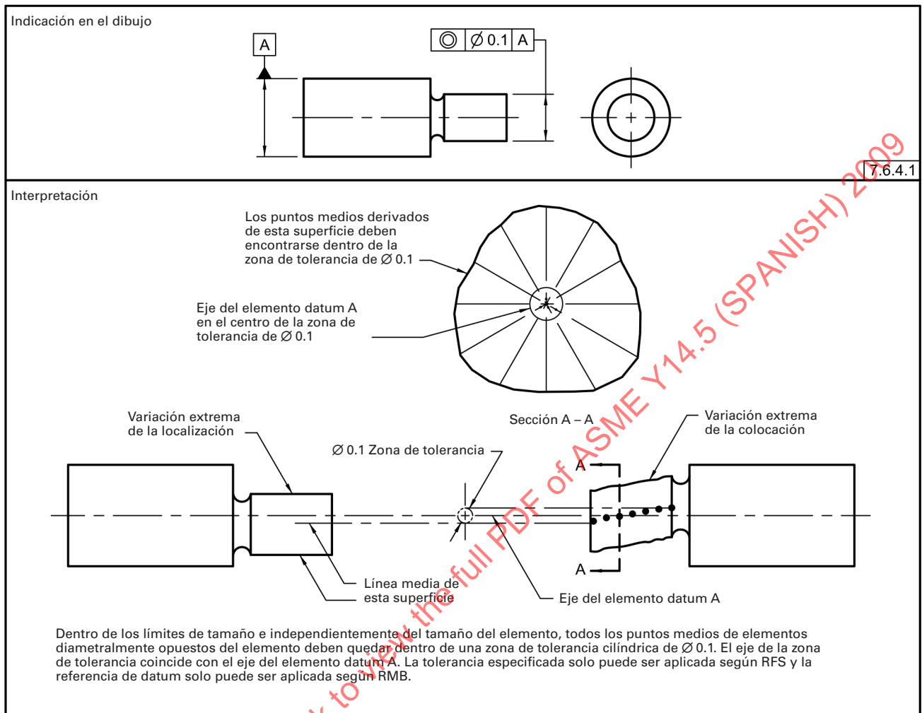
Fig. 7-60 Tolerancia de Concentricidad
