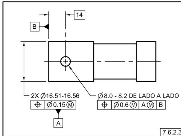
Fig. 7-59 Dos Elementos Datum, Eje Datum Simple
