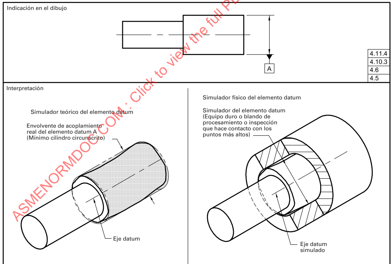
Fig. 4-11 Establecimiento de Datums – Para Elementos Cilíndricos Externos – RMB
