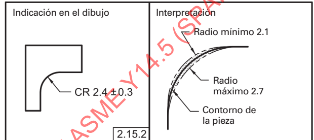
Fig. 2-23 Especificación de un Radio Controlado
