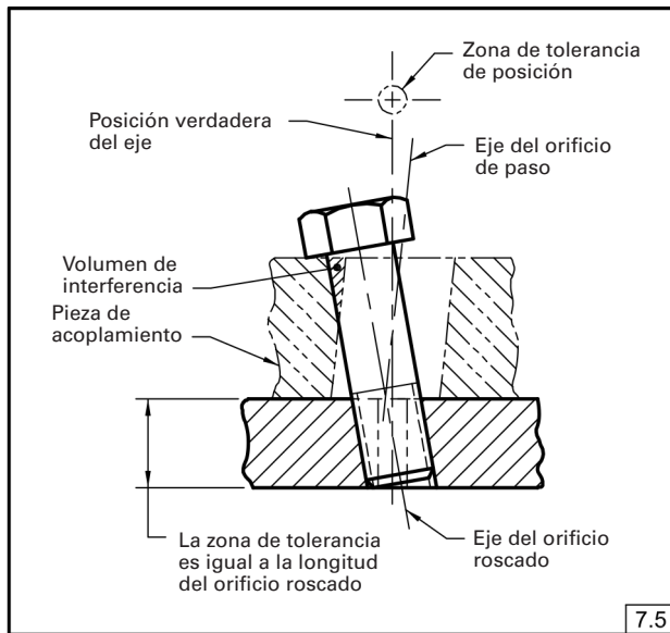
Fig. 7-19 Diagrama de Interferencia, Sujetador y Orificio
