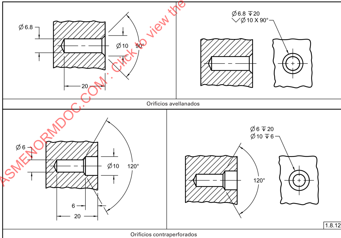
Fig. 1-39 Orificios Avellanados y Contraperforados
