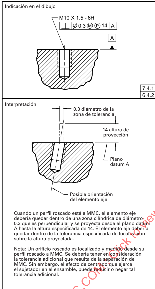
Fig. 6-11 Especificación de la Perpendicularidad para un Eje a una Altura Proyectada (Orificio Roscado o Inserto a MMC)
