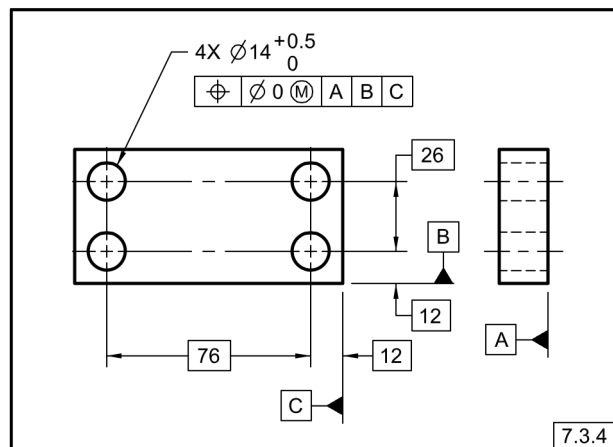
Fig. 7-11 Tolerancia de Posición Cero a MMC
