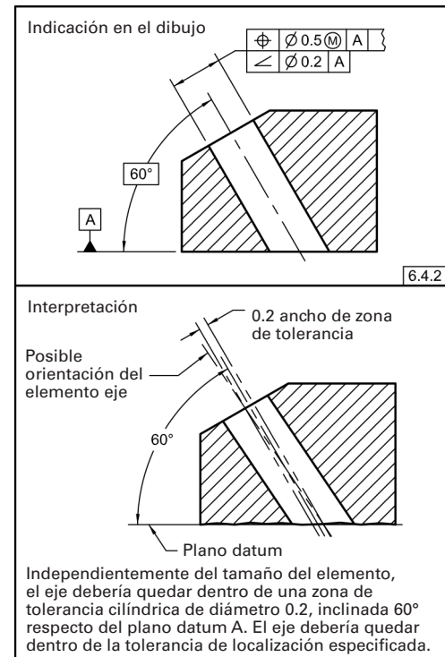
Fig. 6-6 Especificación de la Angularidad para un Eje (Elemento RFS)
