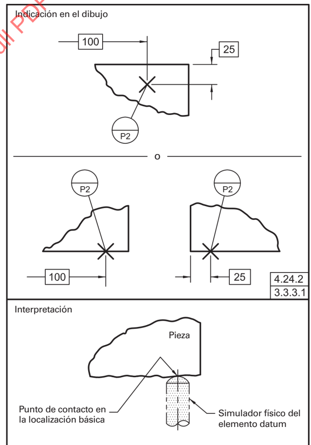
Fig 3-7 Datum objetivo de punto
