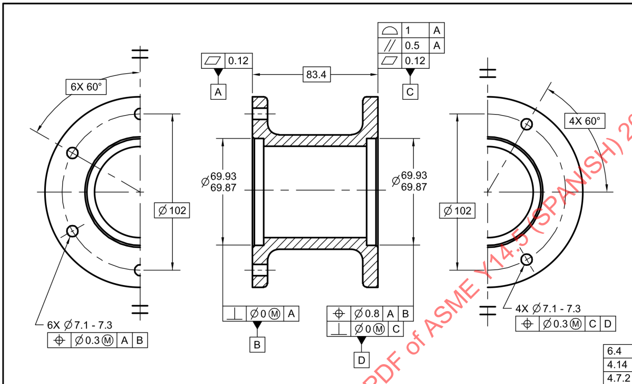
Fig. 4-4 Múltiples Marcos de Referencia Datum y sus interrelaciones
