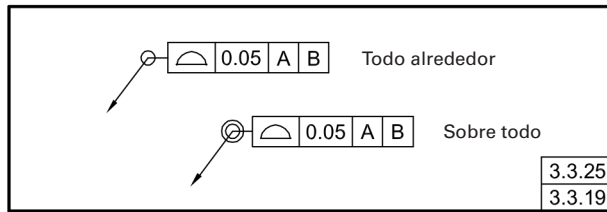
Fig. 3-20 Aplicaciones de Símbolos Todo Alrededor y Sobre Todo
