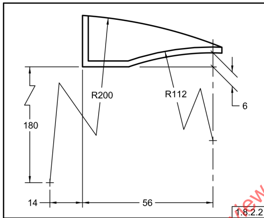
Fig. 1-25 Radios Recortados
