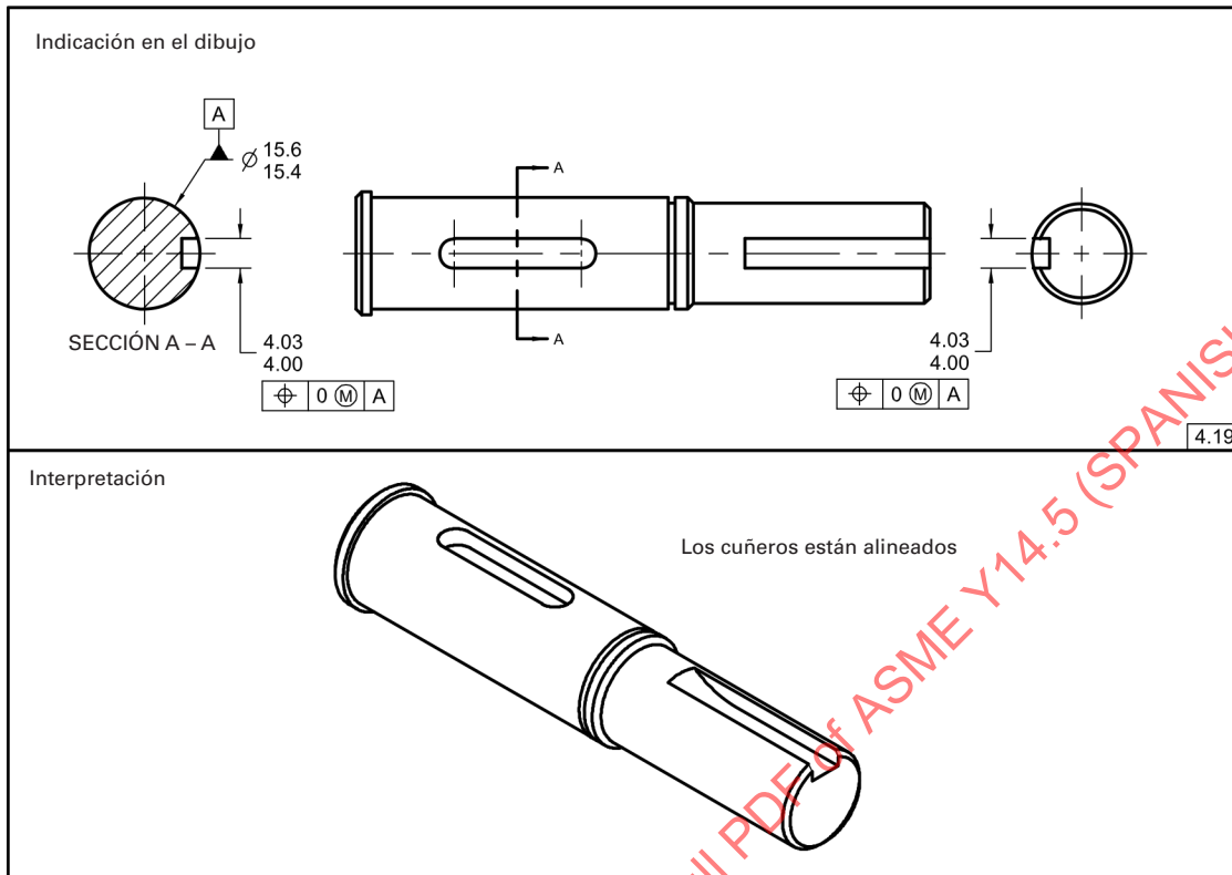
Fig. 4-40 Elementos Alineados – Requerimientos Simultáneos
