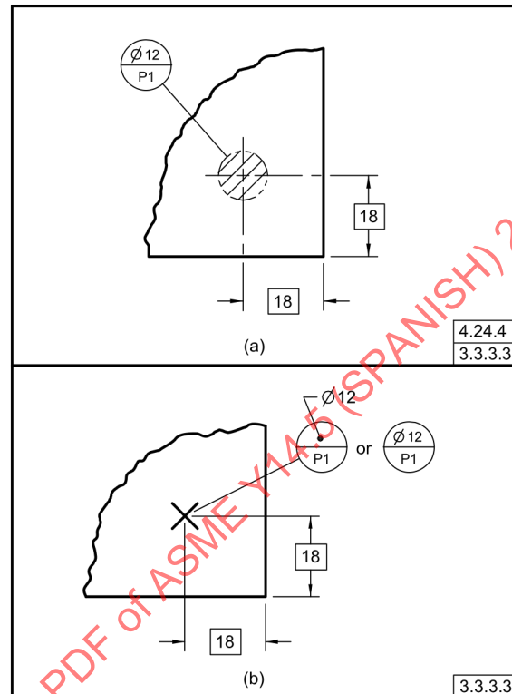
Fig. 3-9 Datum Objetivo de Área
