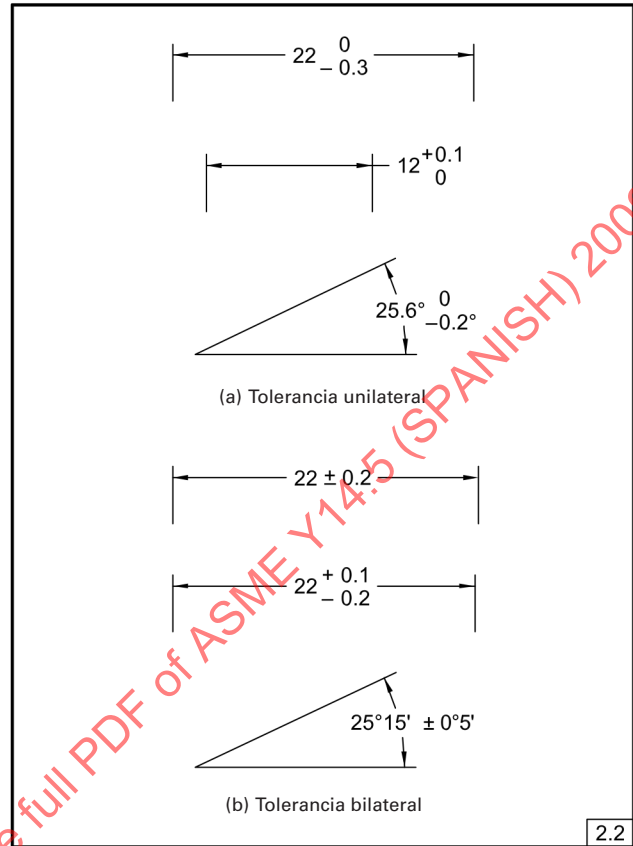
Fig. 2-2 Tolerancia más y menos
