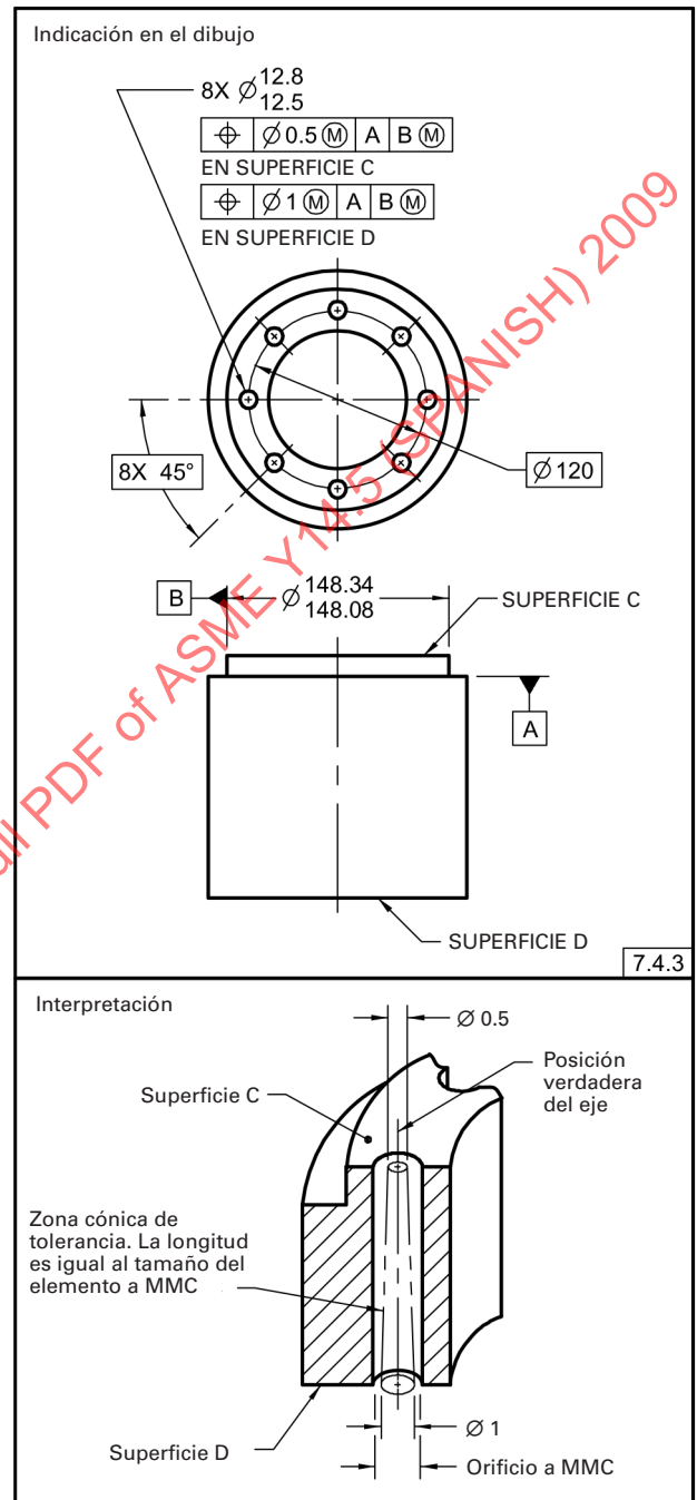
Fig. 7-27 Diferente Tolerancia de Posición para cada Extremo de un Orificio largo
