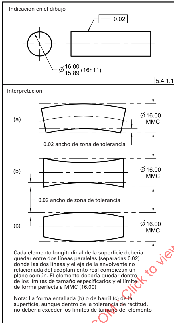
Fig. 5-1 Especificación de la rectitud de elementos de superficie
