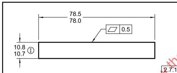
Fig. 2-7 Aplicación de Independencia y Planicidad
