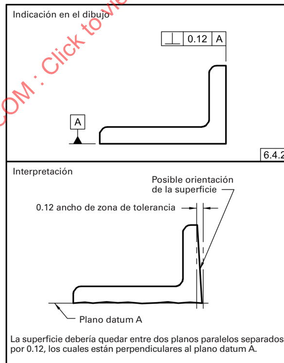
Fig. 6-3 Especificación de la Perpendicularidad para una Superficie Plana
