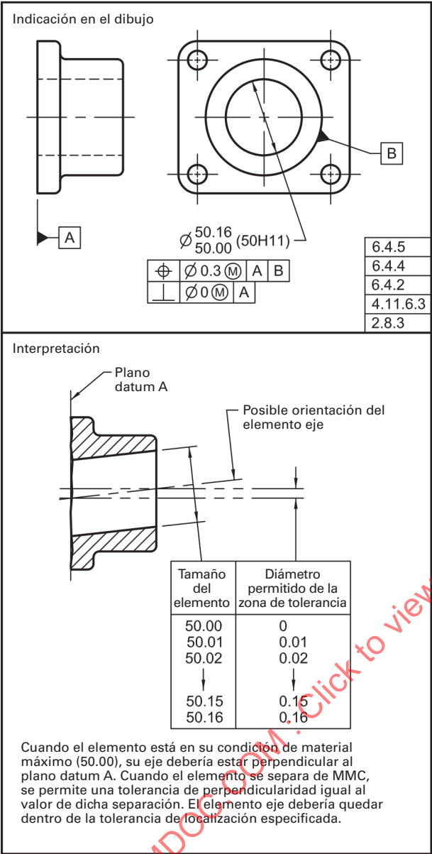
Fig. 6-14 Especificación de la Perpendicularidad para un Eje (Cero Tolerancia a MMC)
