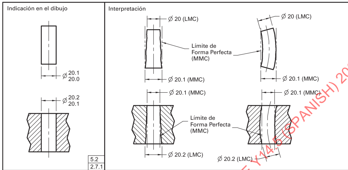
Fig. 2-6 Variaciones Extremas de Forma Permitidas por una Tolerancia de Tamaño
