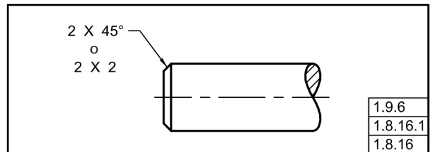
Fig. 1-43 Chaflán de 45°
