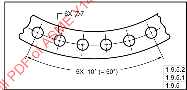
Fig. 1-56 Elementos y Dimensiones Repetitivos
