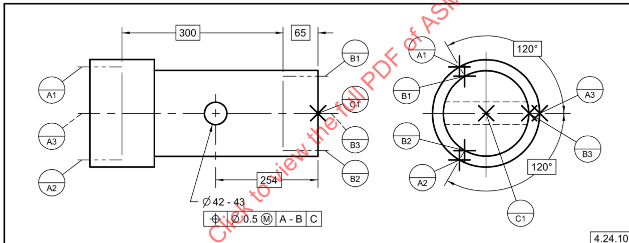
Fig. 4-51 Datums Primario y Secundario Establecidos por Datum Objetivo por Líneas en dos Elementos Cilíndricos y una Superficie
