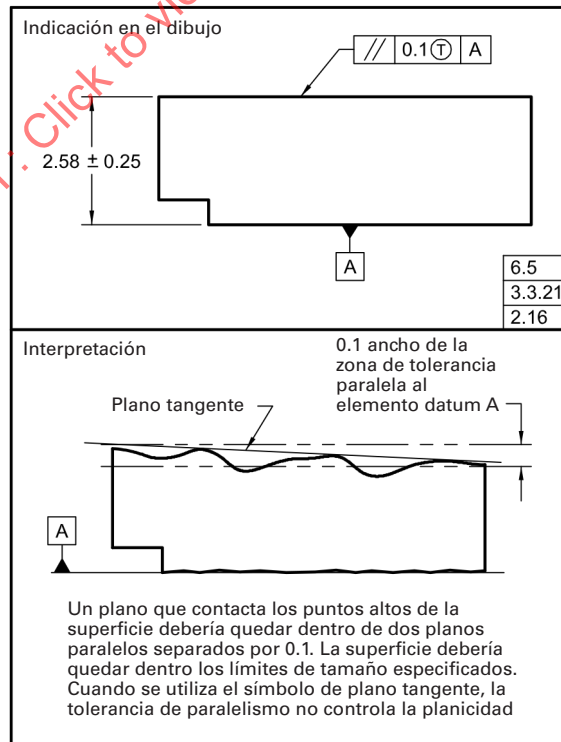
Fig. 6-18 Especificación de un Plano Tangente
