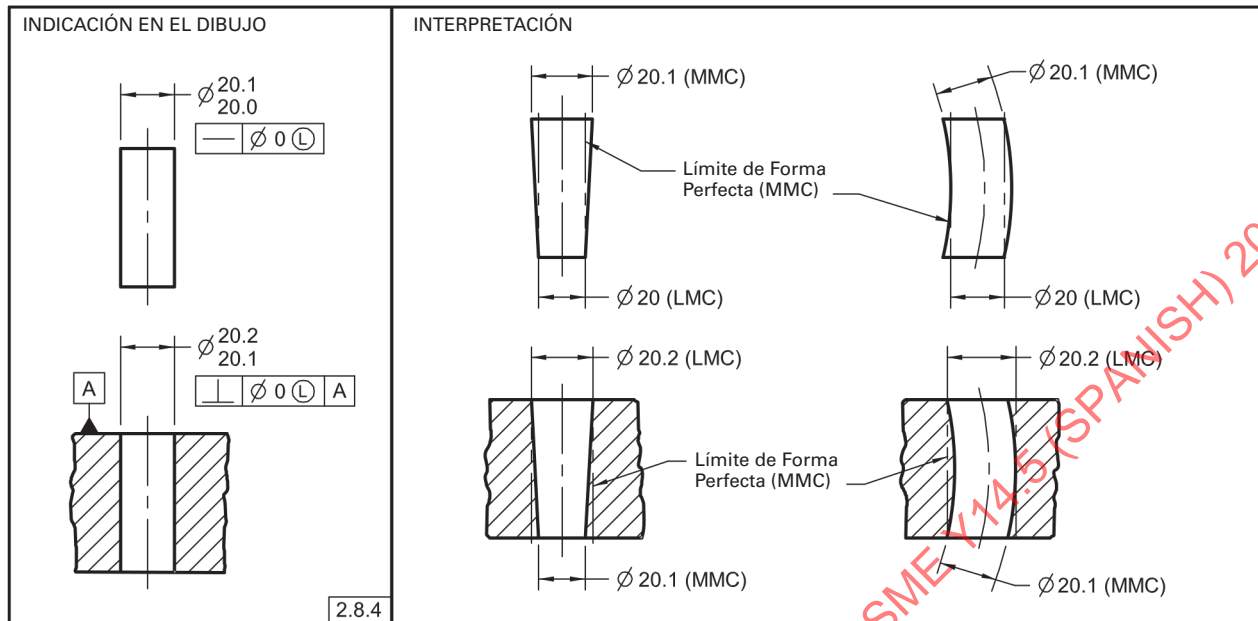
Fig. 2-11 Variaciones Extremas de Forma Permitidas por una Tolerancia Geométrica – Forma Perfecta en LMC
