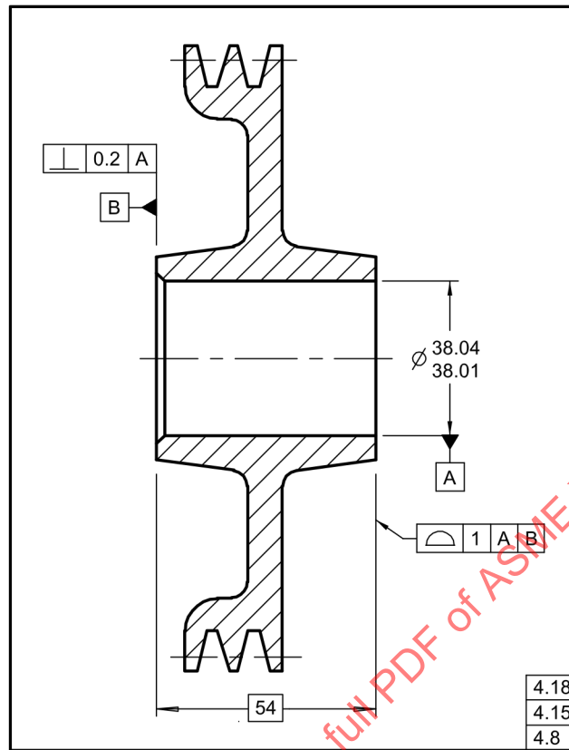
Fig. 4-37 Aplicación de Datum Funcional – Polea
