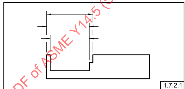
Fig. 1-11 Líneas de Extensión Interrumpidas
