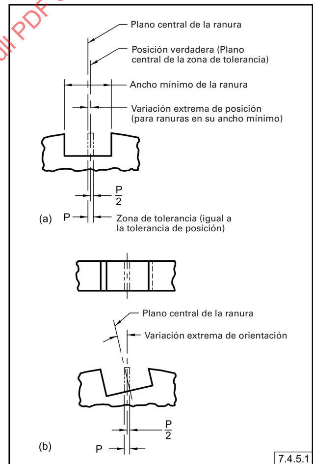
Fig. 7-33 Zona de Tolerancia para Planos Centrales de Ranuras a MMC
