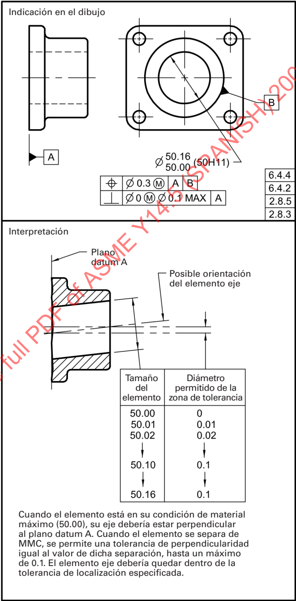
Fig. 6-15 Especificación de la Perpendicularidad para un Eje (Cero Tolerancia a MMC con un Máximo Especificado)
