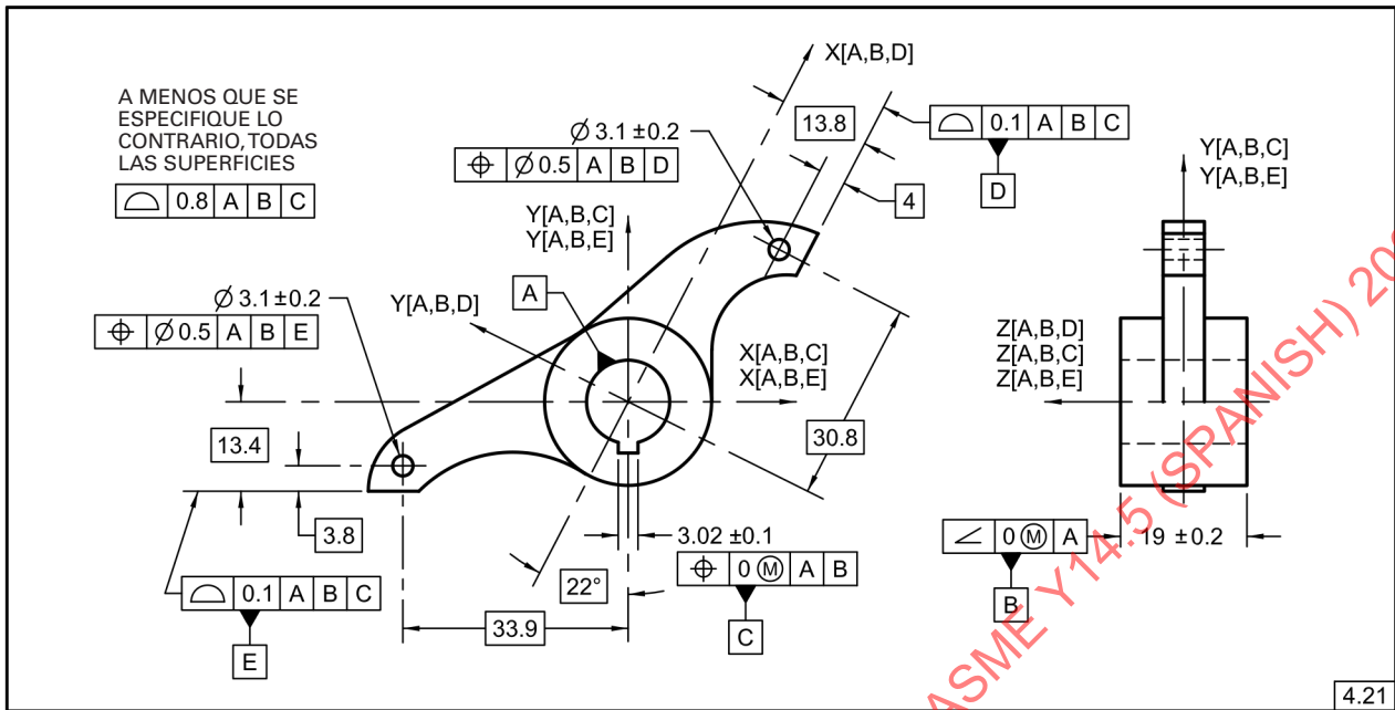
Fig. 4-43 Identificación del Marco de Referencia Datum
