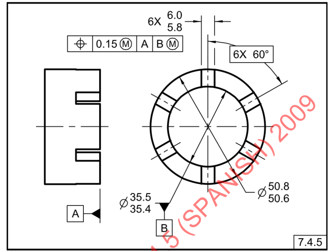
Fig. 7-31 Tolerancia de Posición de Ranuras
