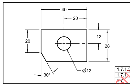
Fig. 1-6 Aplicación de Dimensiones
