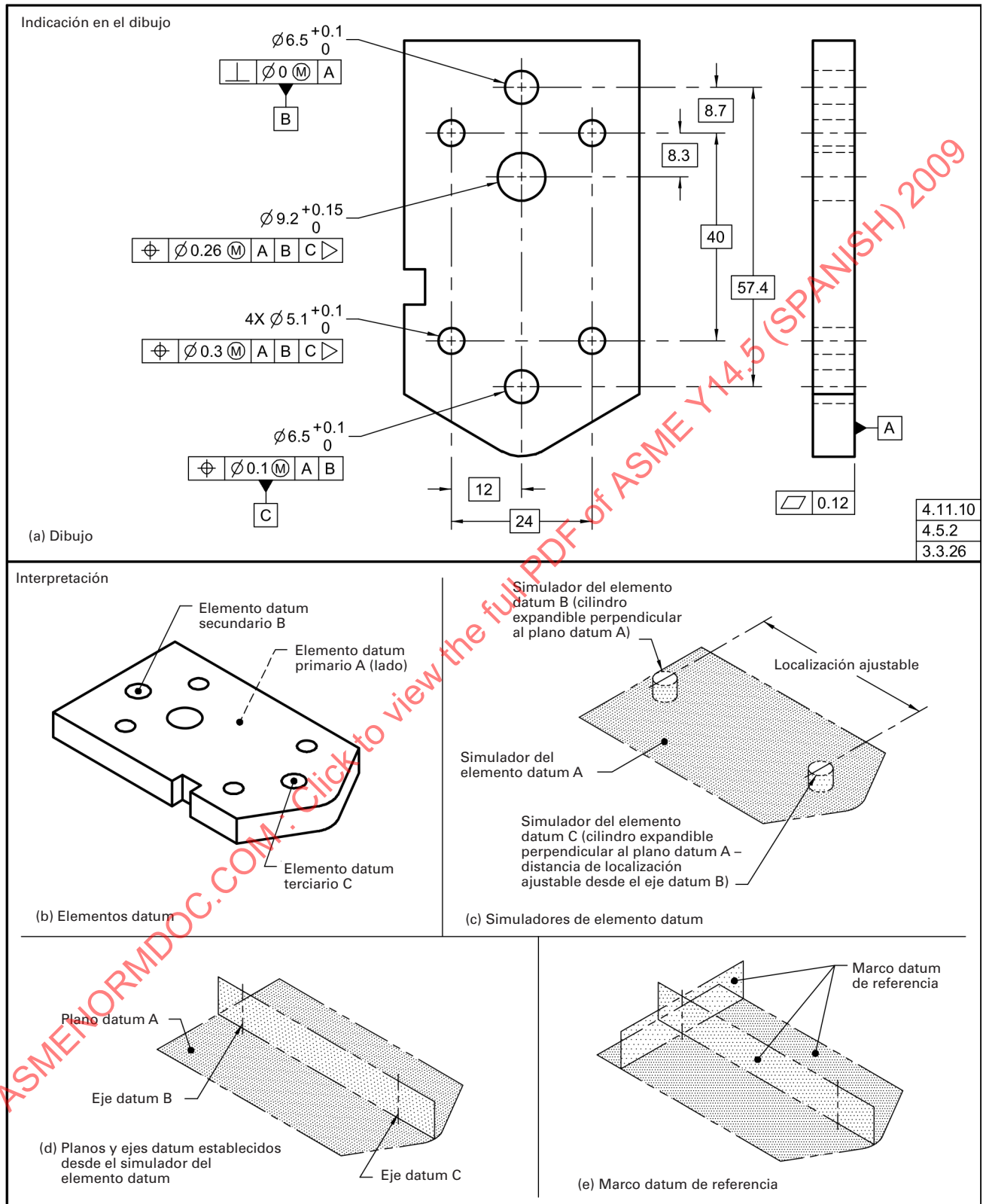
Fig. 4-19 Desarrollo de un Marco Datum de Referencia con Modificador de Traslación
