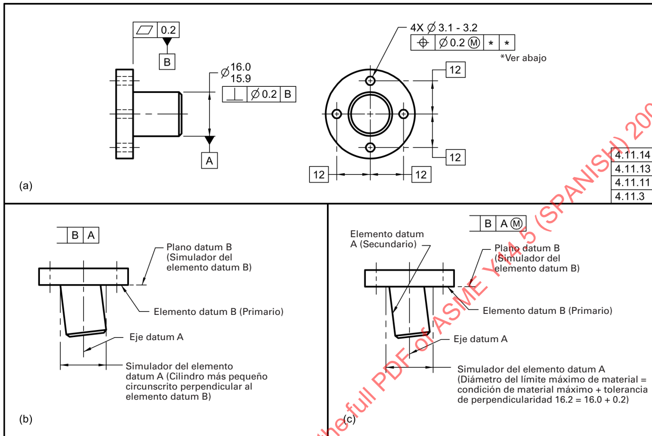
Fig. 4-20 Efecto del Modificador Datum
