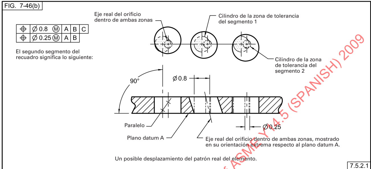
Fig. 7-46 Patrones de Orificios de la Fig. 7-46. Marcos de Control de Elemento de Múltiples Segmentos Individuales con Datum Secundario en el Marco de Control de Elemento Inferior (Continuación) (Límites de Aceptación para orificios en el Patrón)
