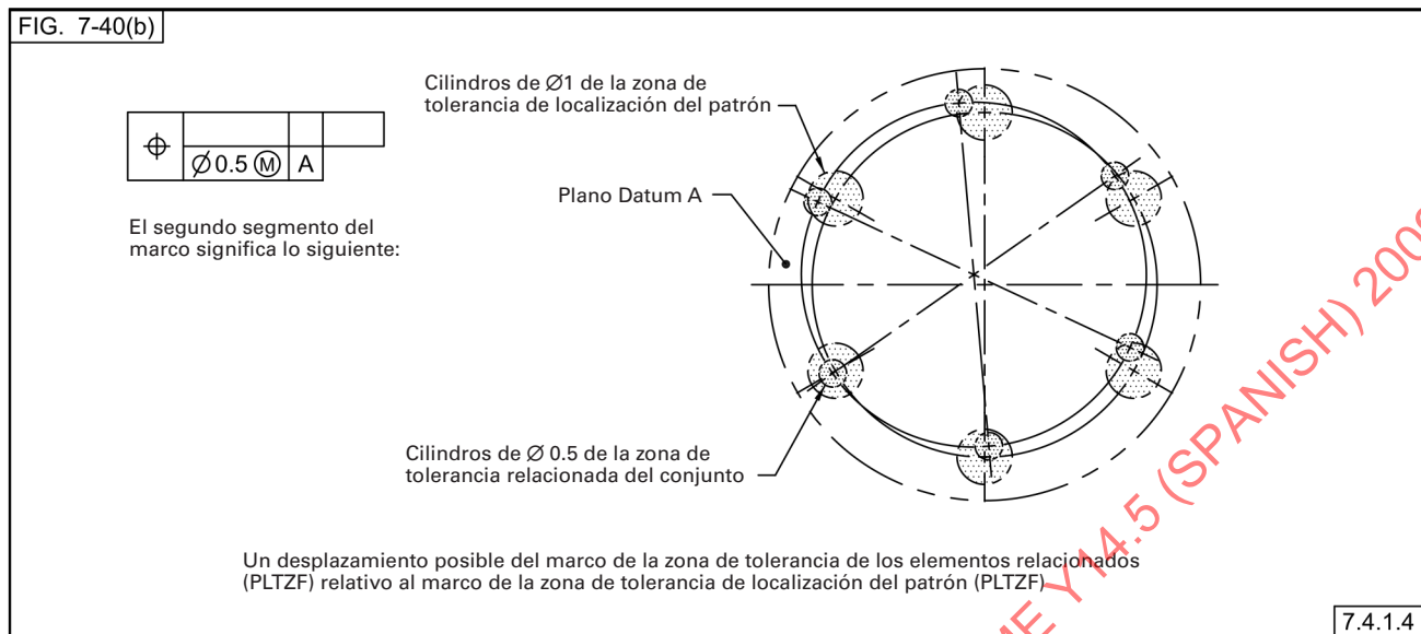
Fig. 7-40 Tolerancia Compuesta de Posición de un Patrón Circular de Elementos (Continuación)
