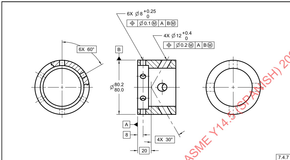
Fig. 7-36 Orificios No Paralelos Incluidos Aquellos No Normales a la Superficie
