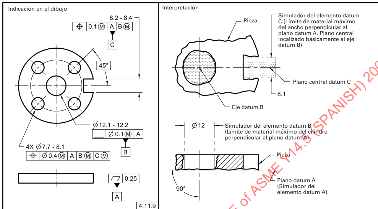
Fig. 4-18 Elementos Datum Secundario y Terciario a MMB
