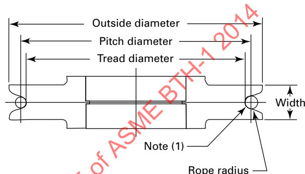
Fig. 4-2.6-1 Sheave Dimensions
