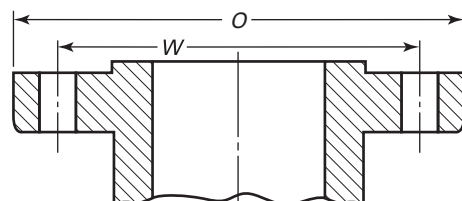
Flange
